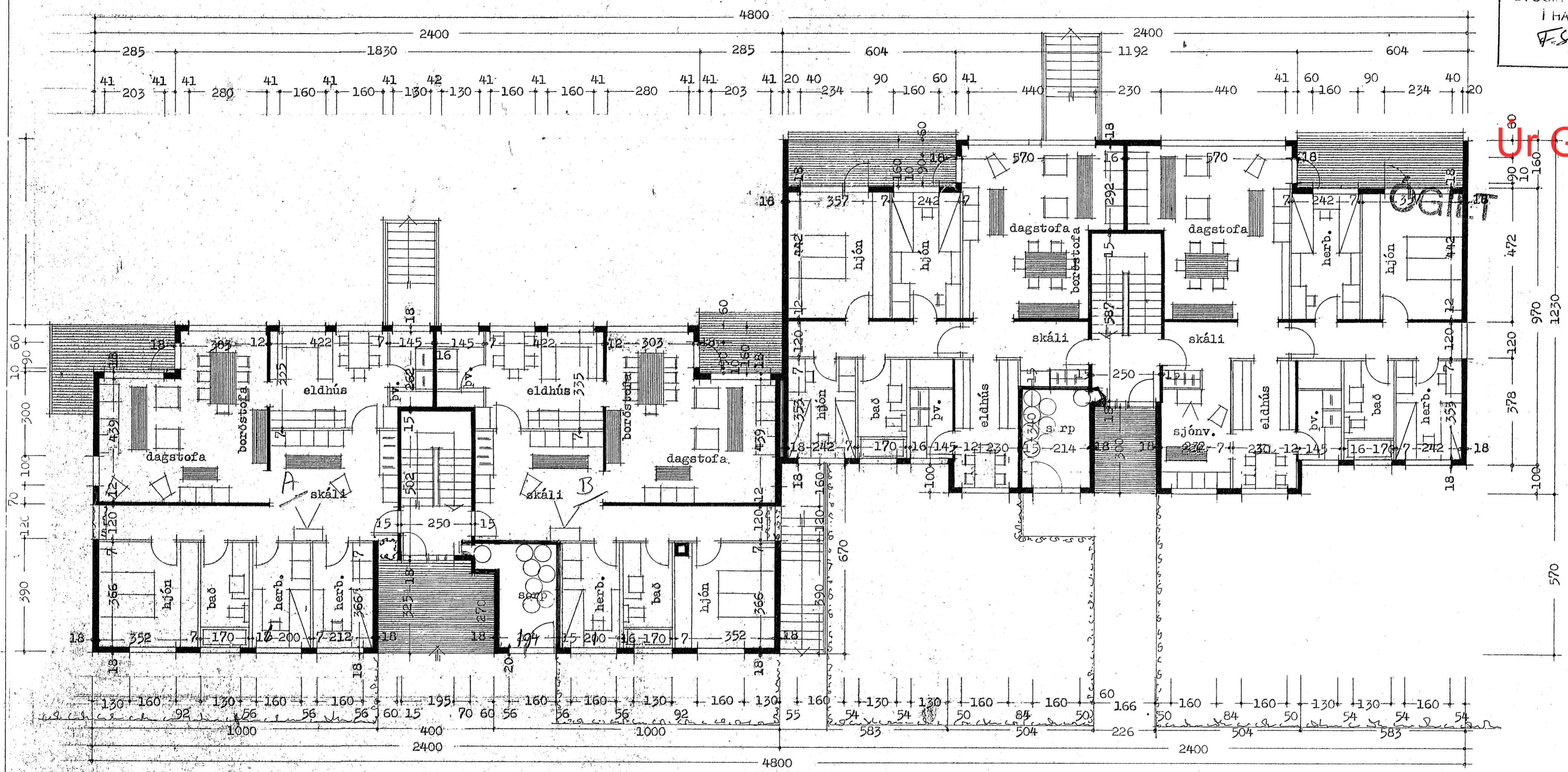
grunnmynd 1. hæð
