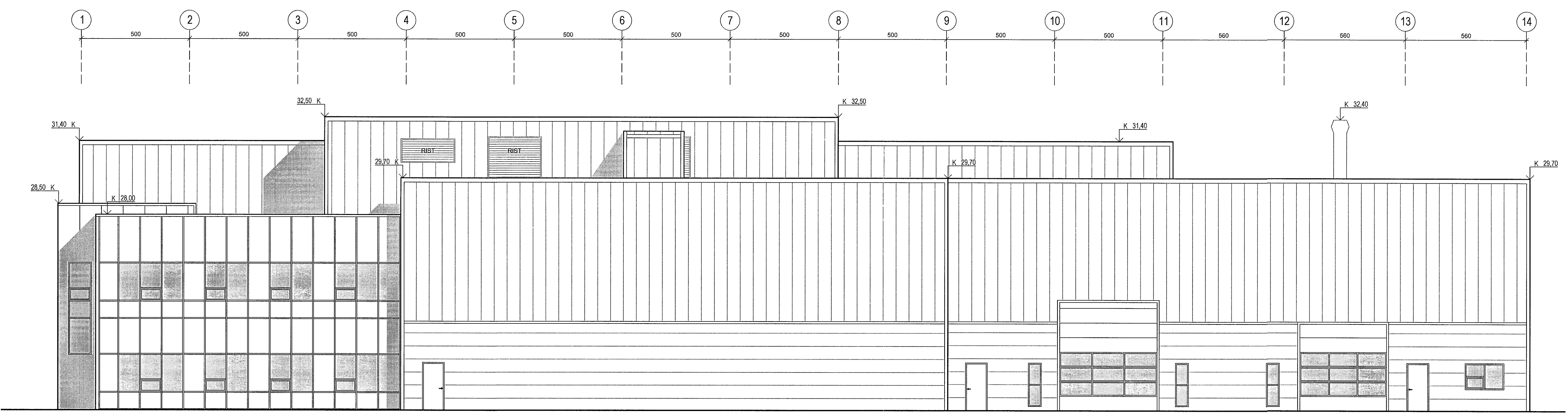
1 ÚTLIT 1:100 ÚTLIT VESTUR
