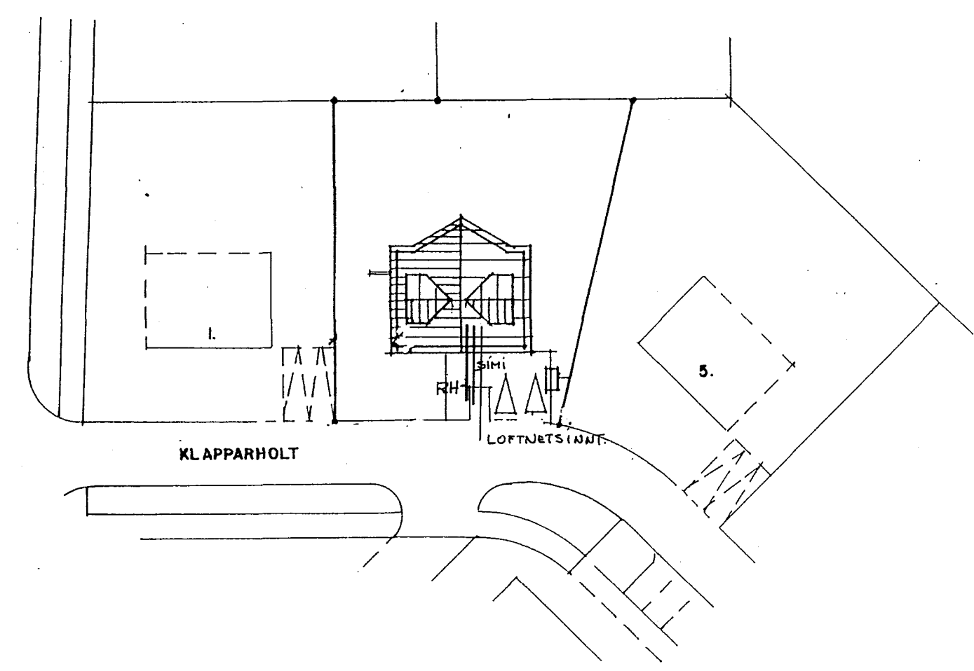
AFSTÖÐUMYND M. 1:500
