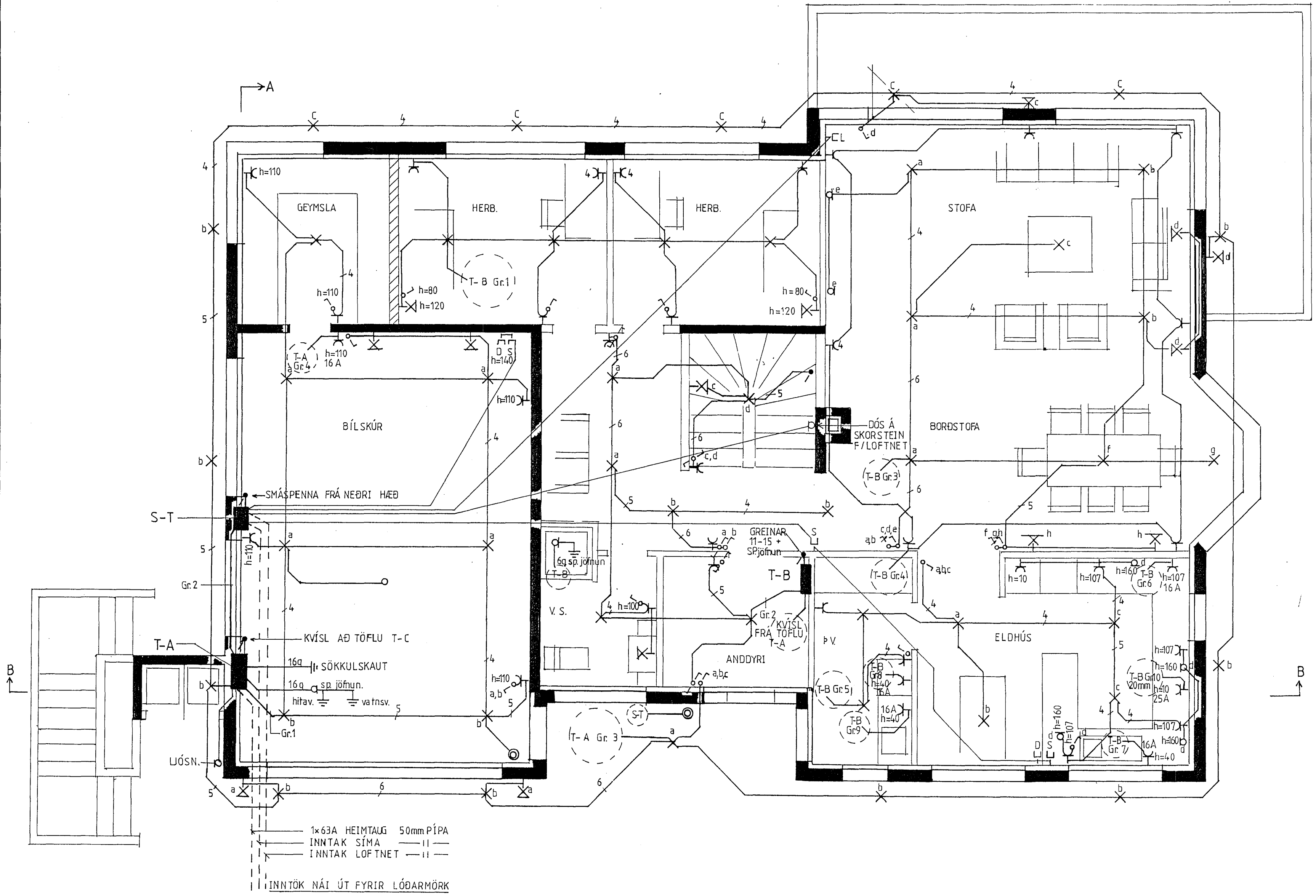
GRUNNMYND EFRI HÆÐAR MKV. 1:50
