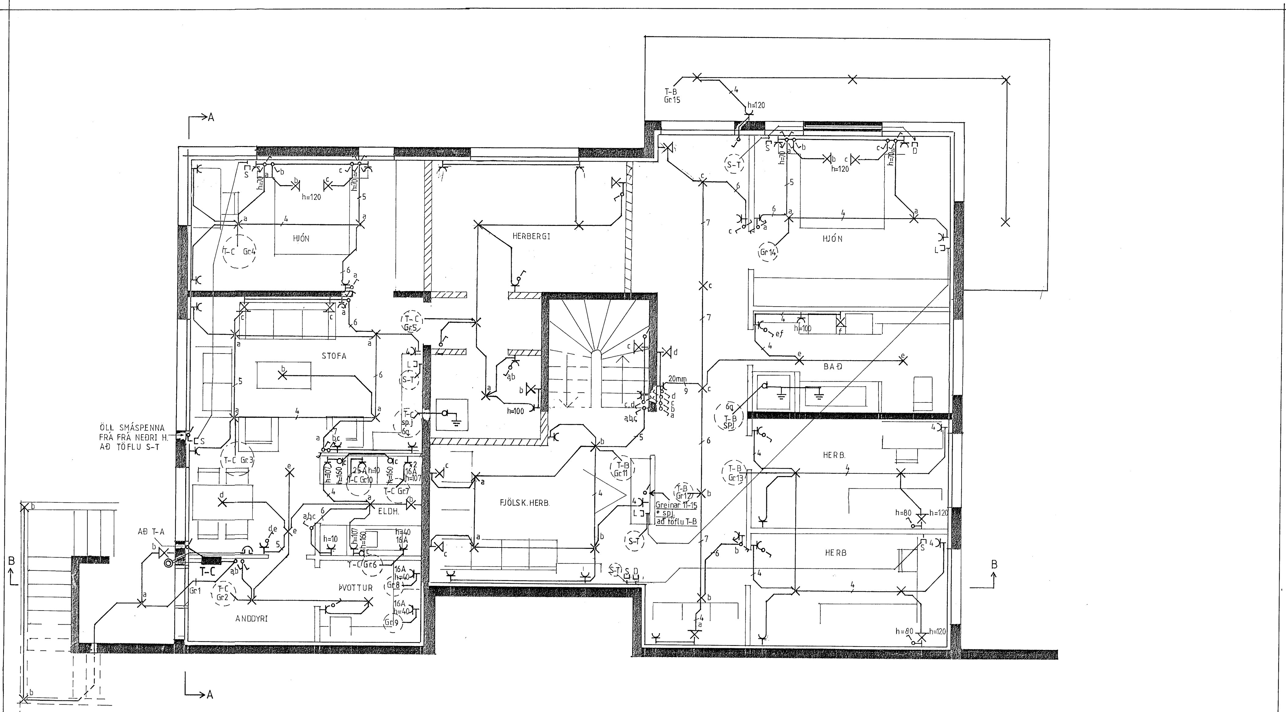
GRUNNMYND NEÐRI HÆÐAR MKV. 1:50
