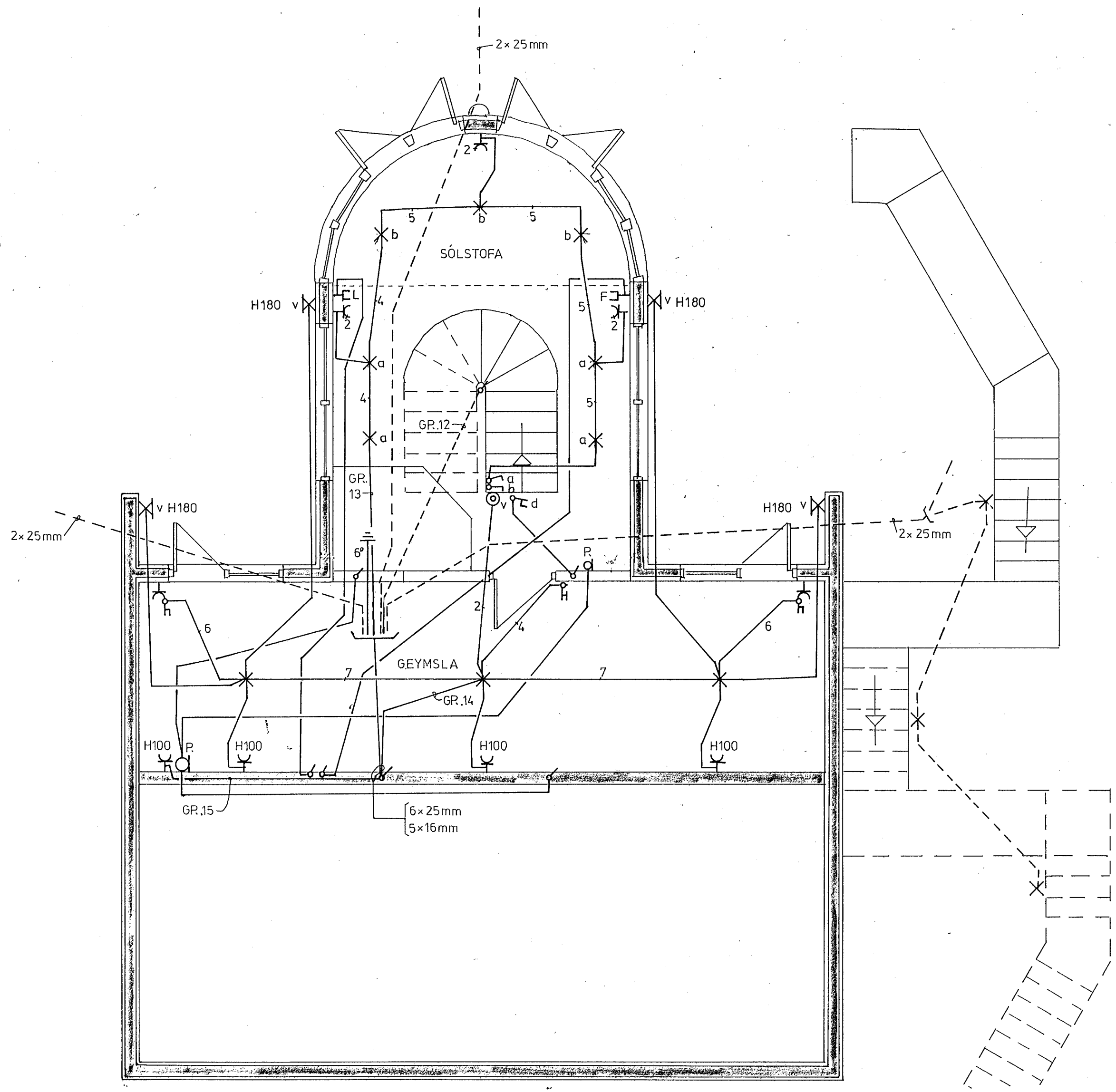
LÁG- OG SMÁSPENNA KJALLARA M1:50
