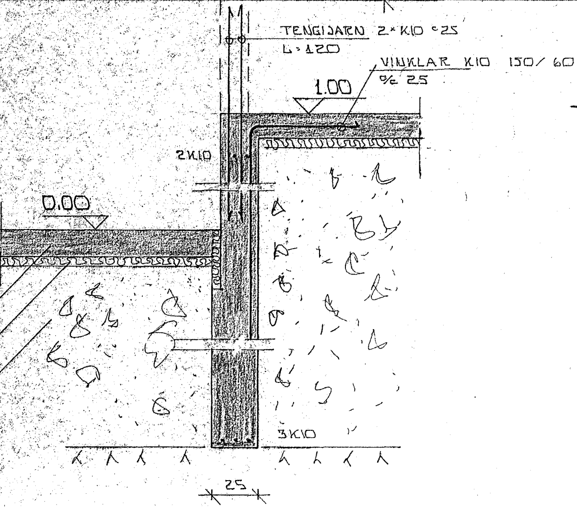
SNIB I VEGG MED HEDARMISMUN 1:20
