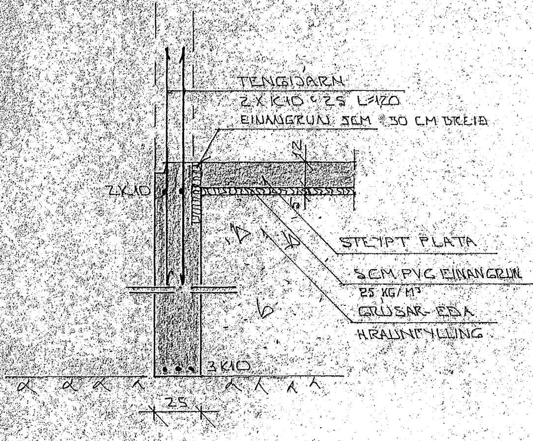
SNIB I UTVEGG 1:20
