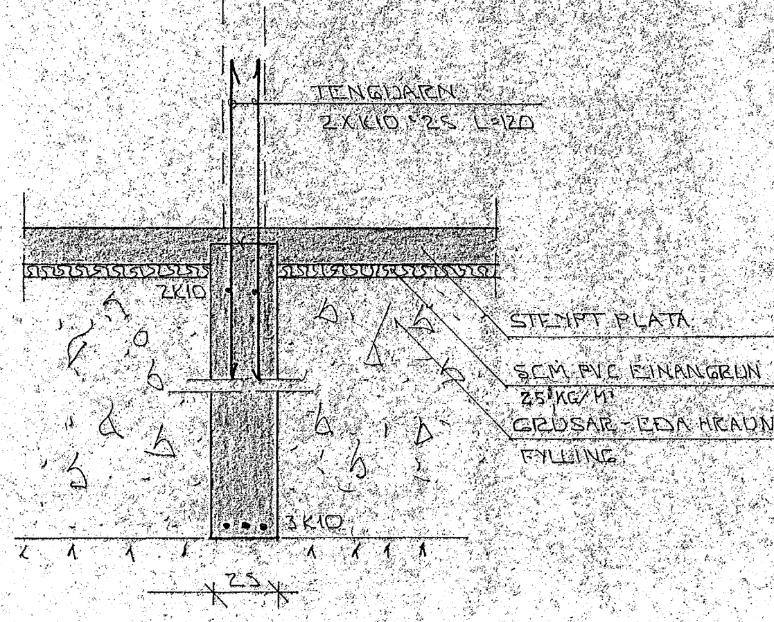
SNIB I INNVEGG 1:20
