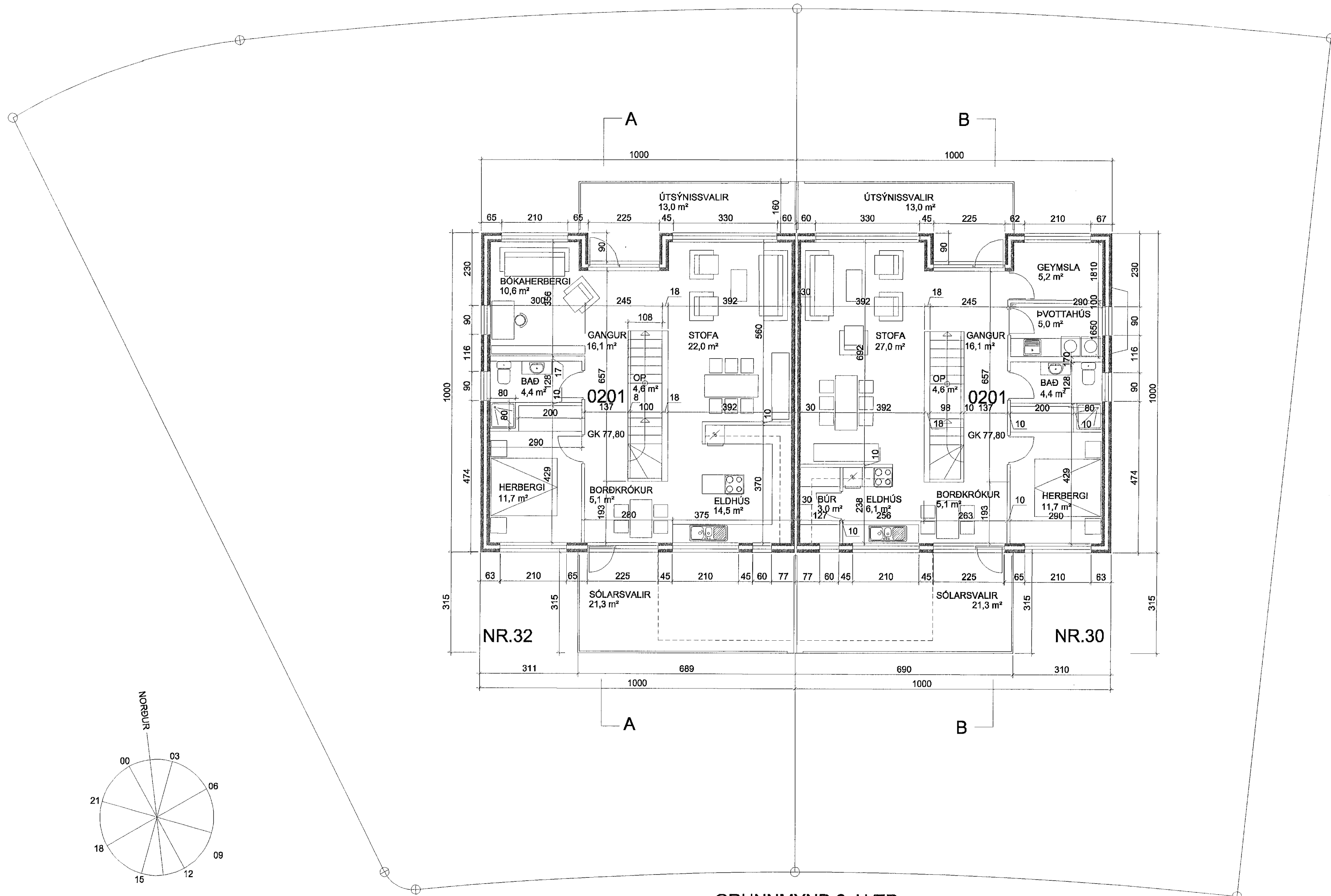
GRUNNMYND 2. HÆÐ
