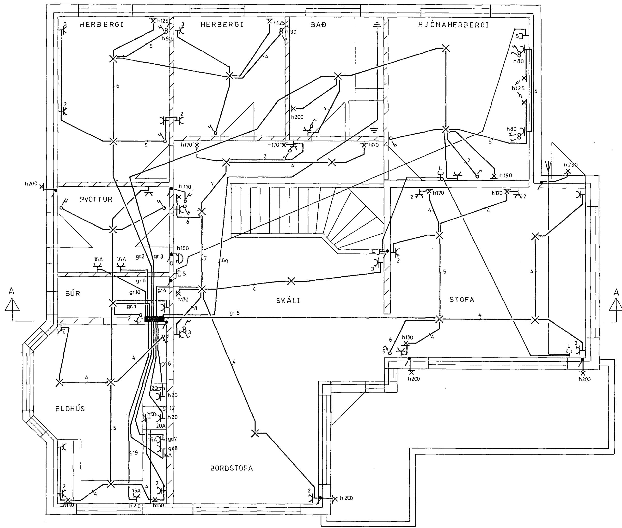
GRUNNMYND 2. HÆÐ M1:50
