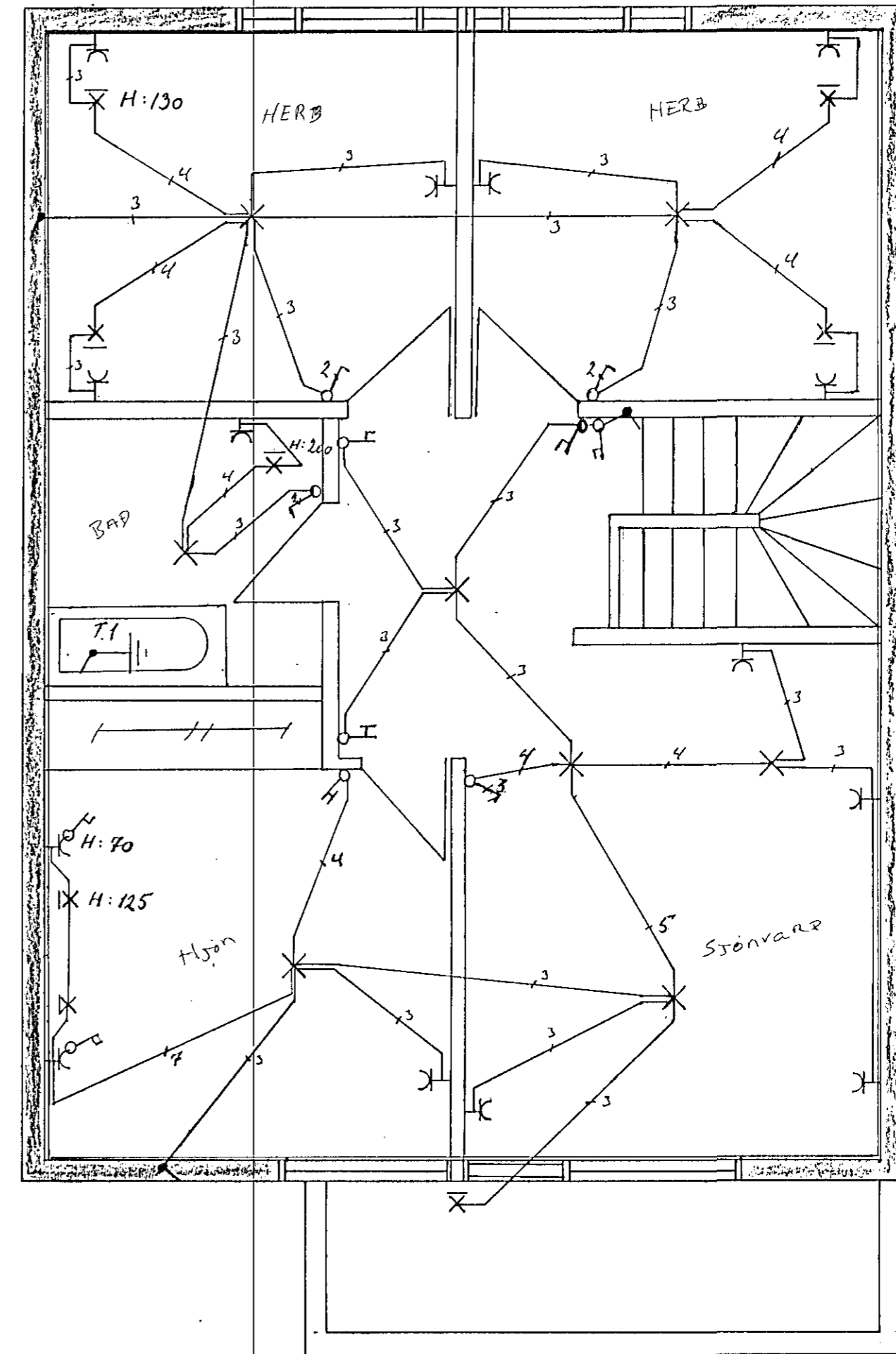
2. HÆÐ
