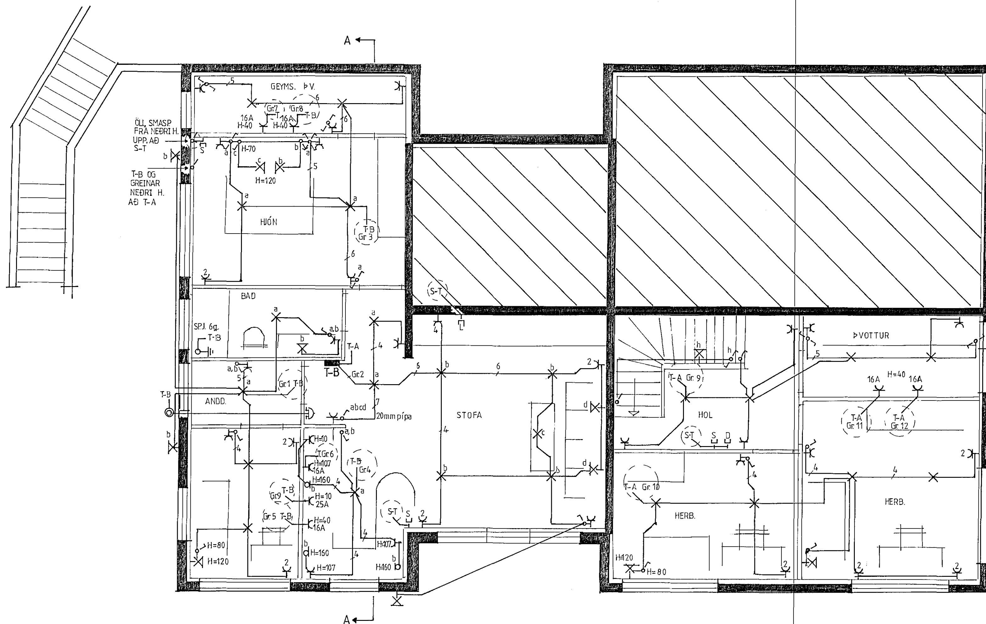
GRUNNM. JARÐH. M=1:50
