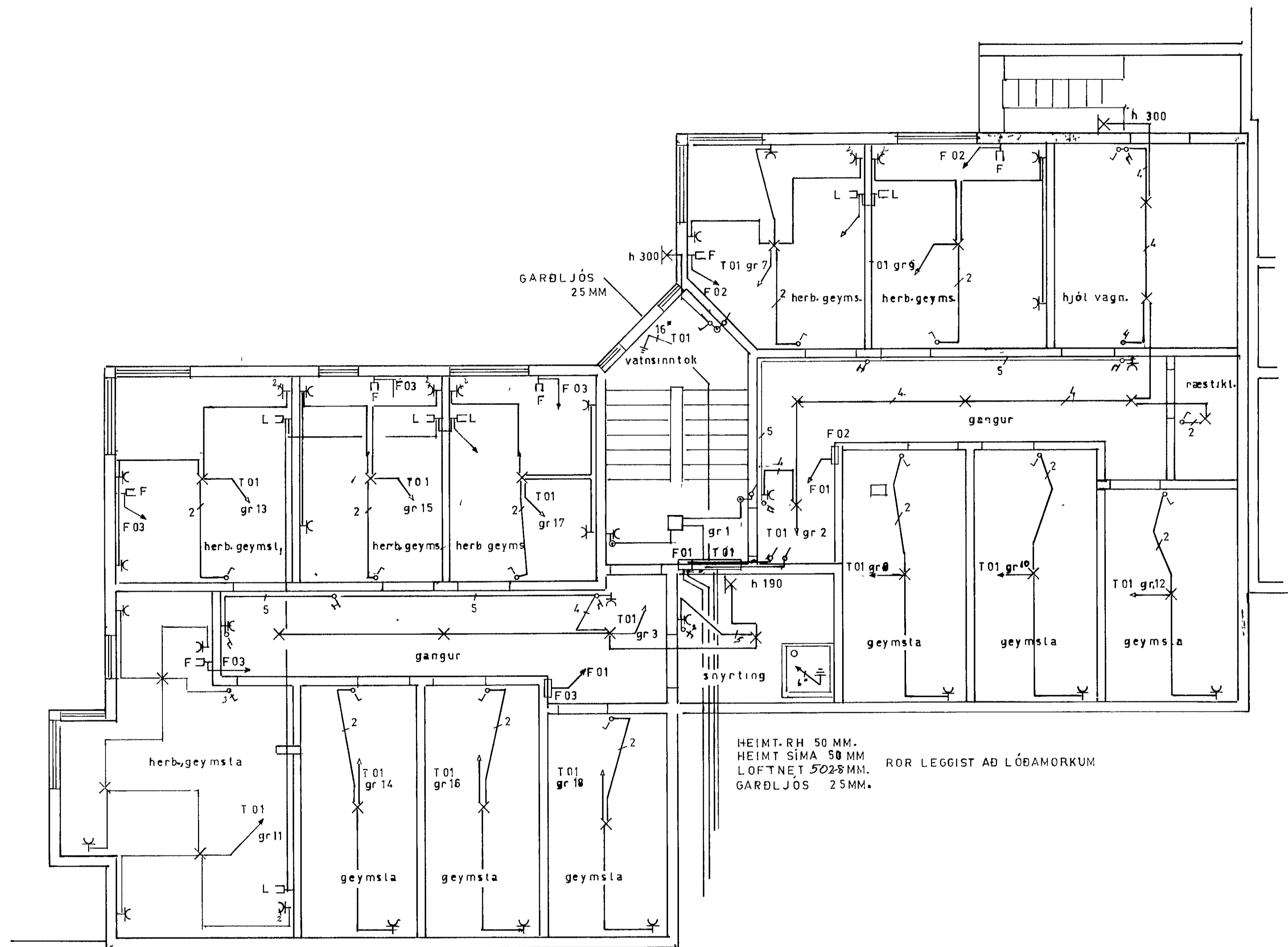
grunnmynd kjallara 1:50
