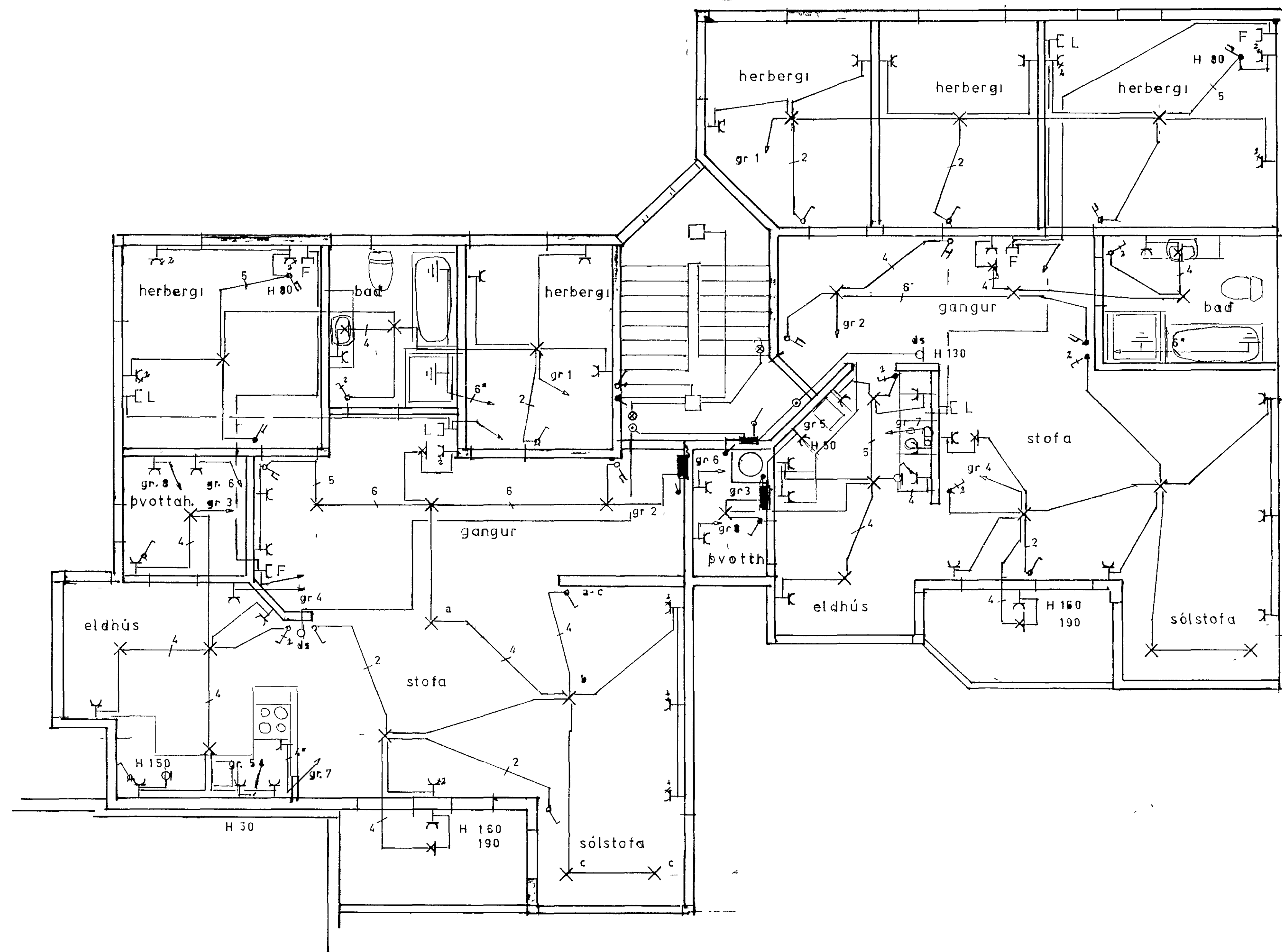
GRUNNMYND 2 hæð 1:50
