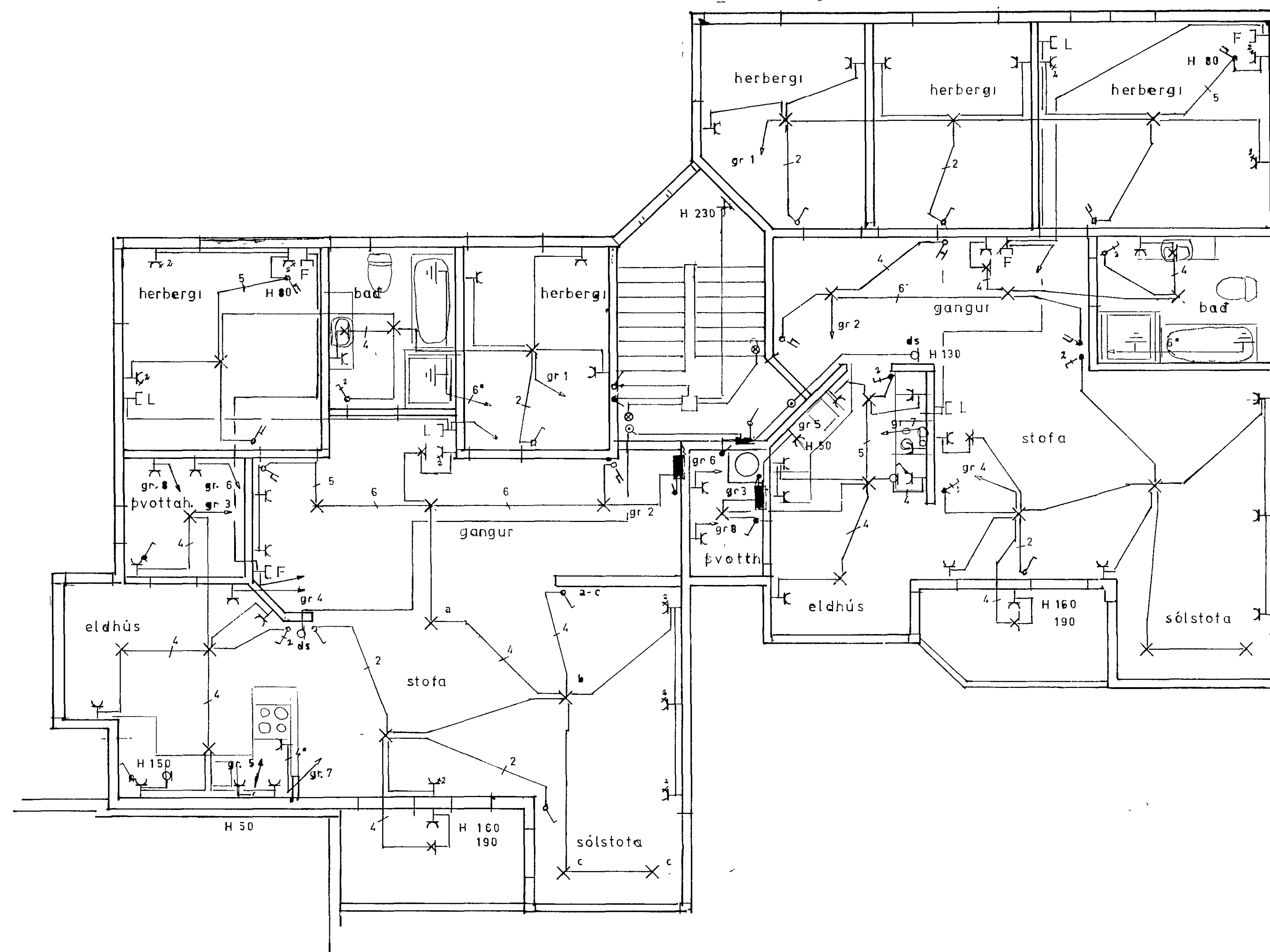
GRUNNMYND 3. hæð 1:50
