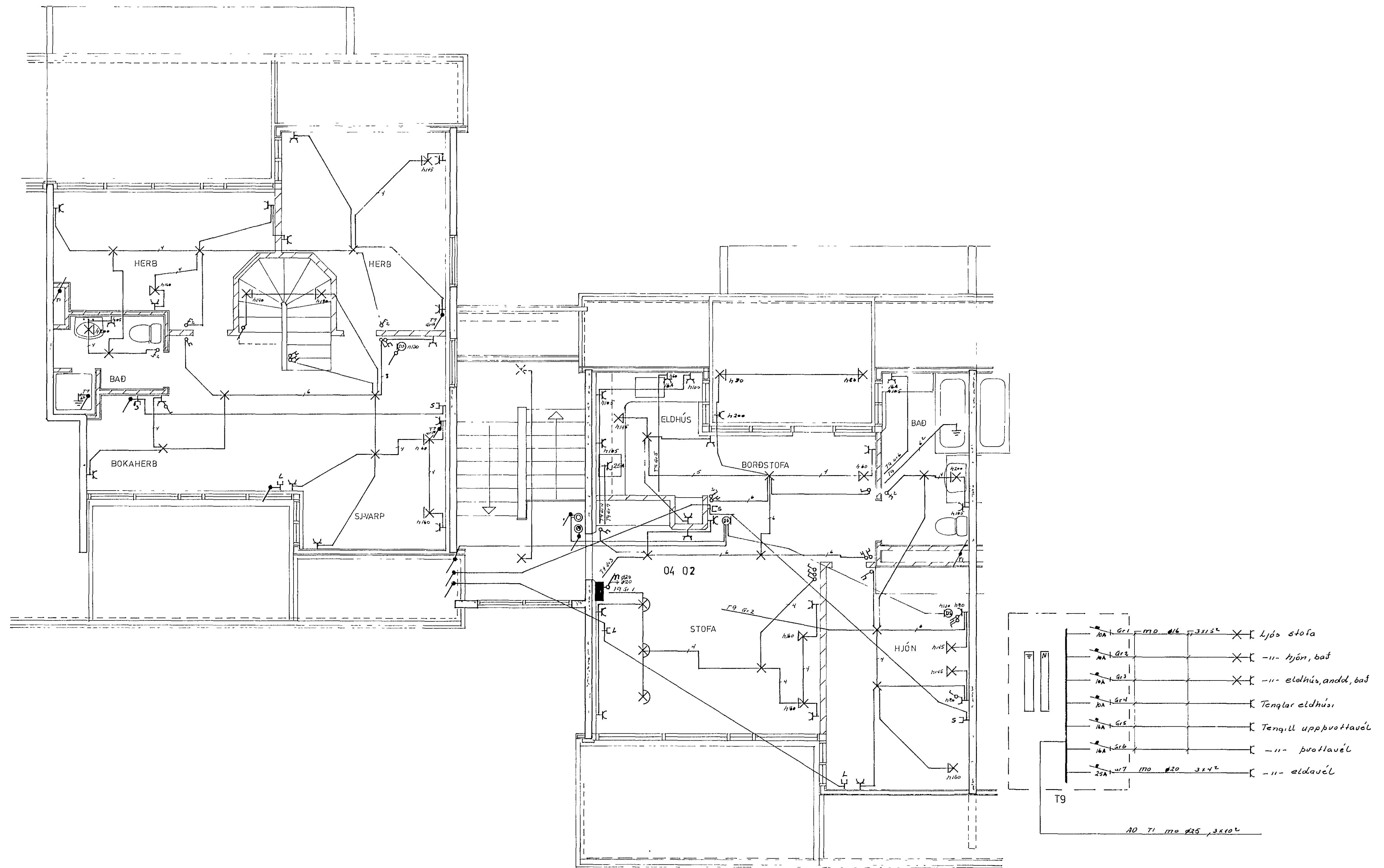
GRUNNMYND 4 HÆÐAR
