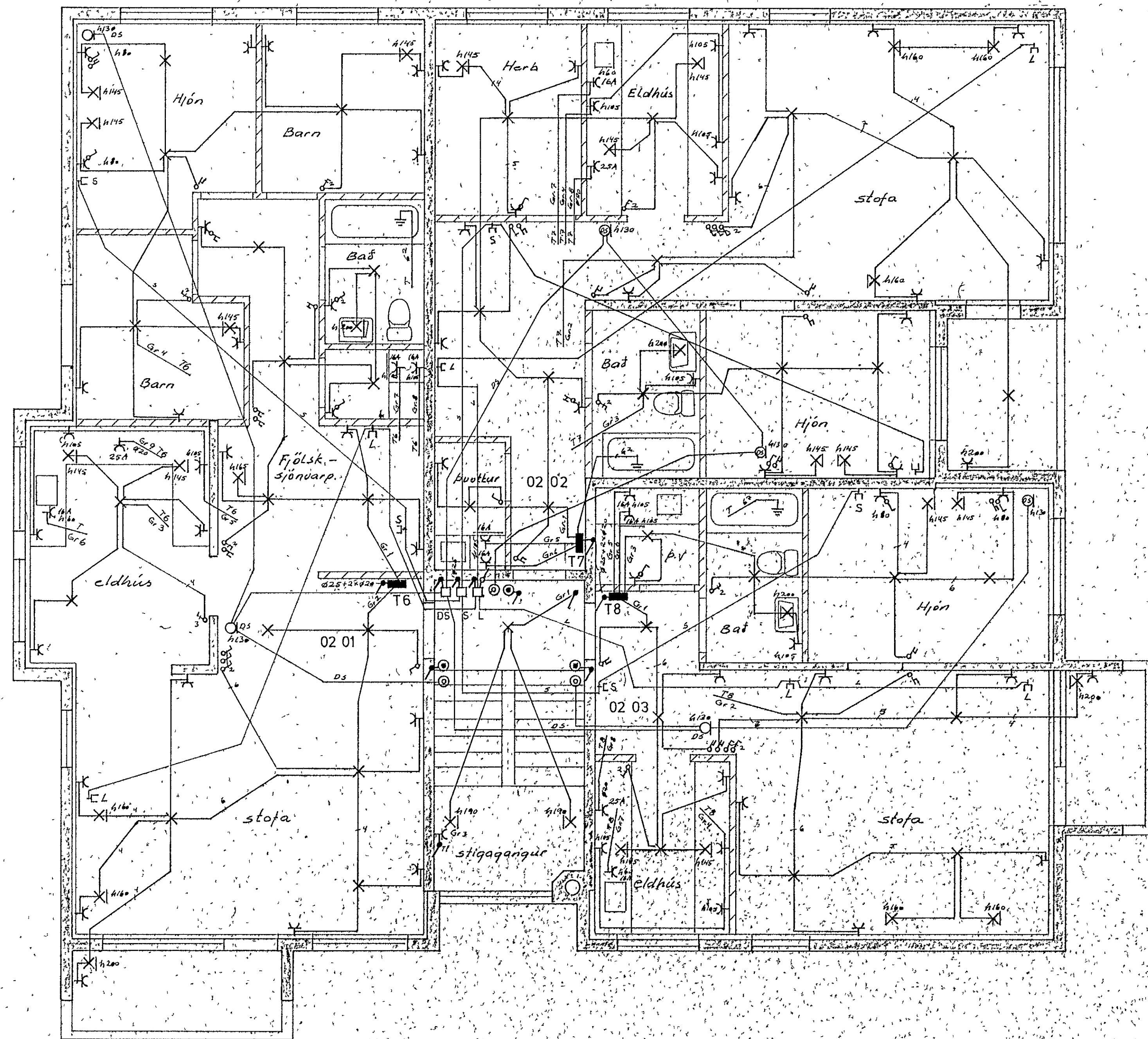
GRUNNMYND 2 HÆÐAR M. 1:50
