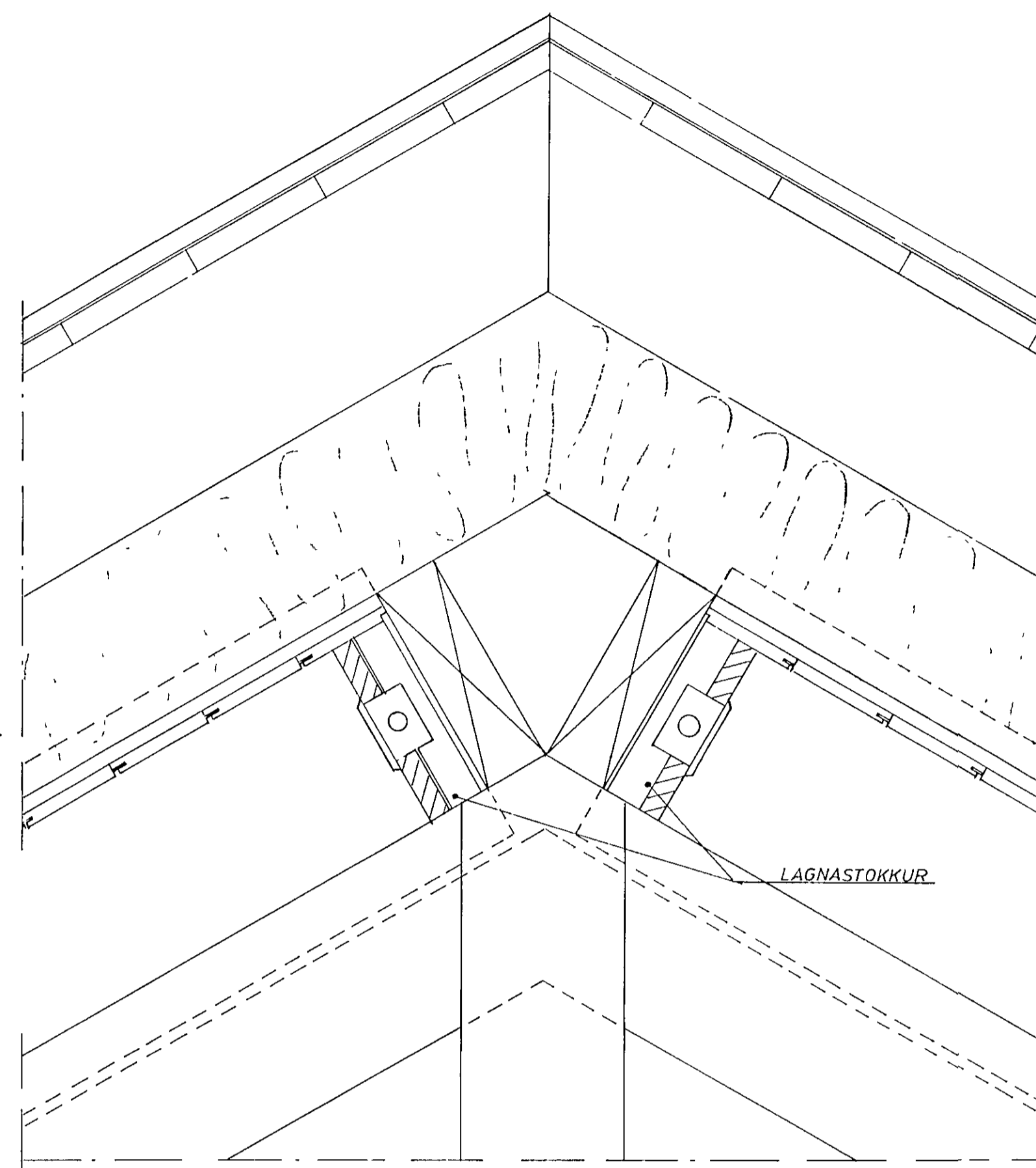
SNID A-A M. 1:5
