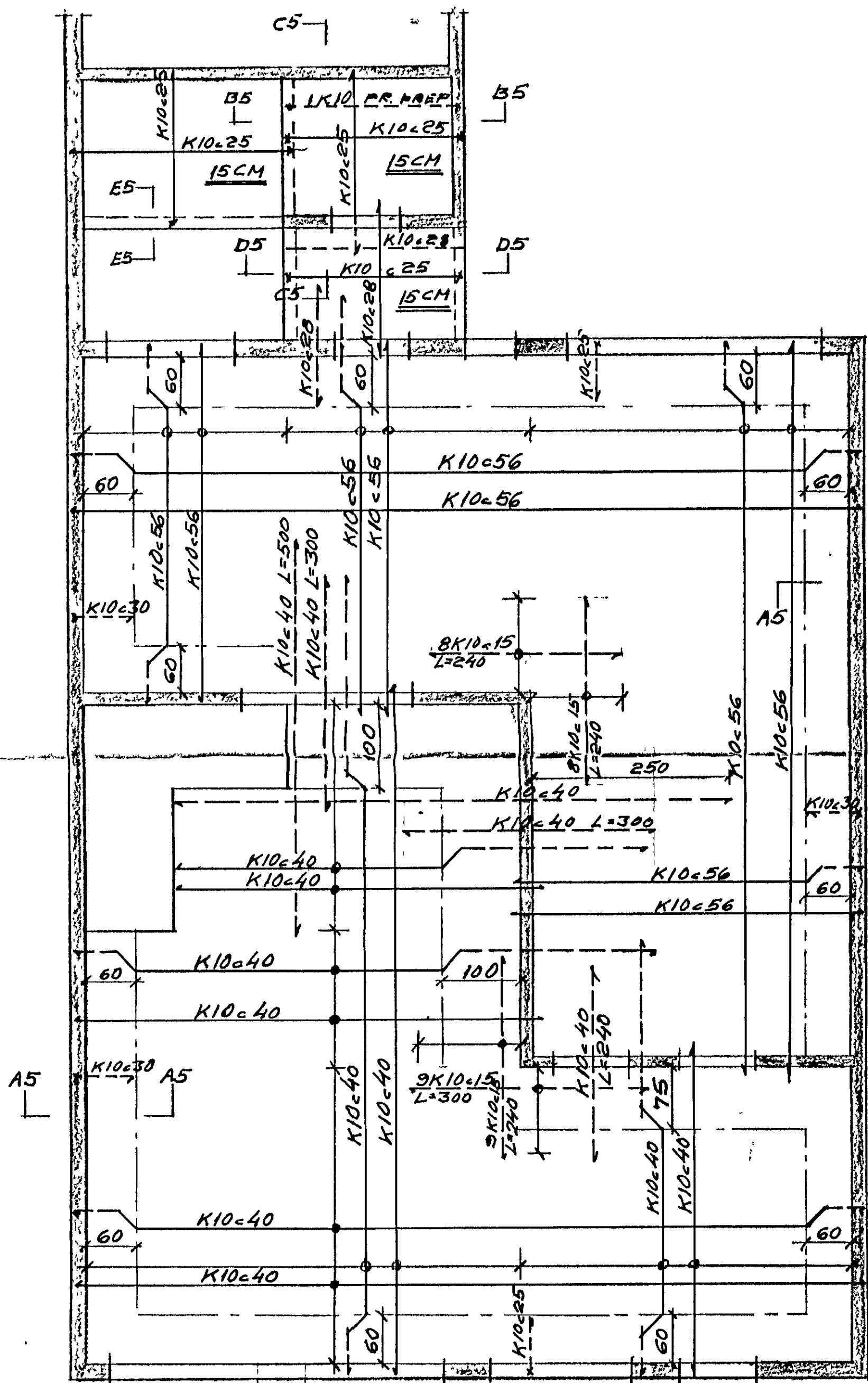
KJALLARALOFT I NR. 3 PLÖTUR 20CM -1:50-
