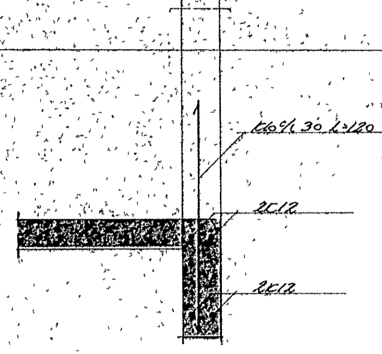
SNID B-B 1:20
