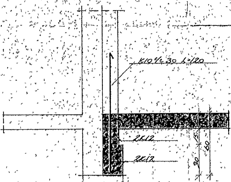
SNID A-A 1:20
