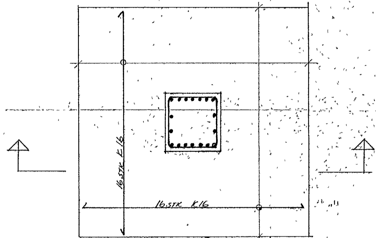
UNDIRSTÖÐA 1-1 1:20
