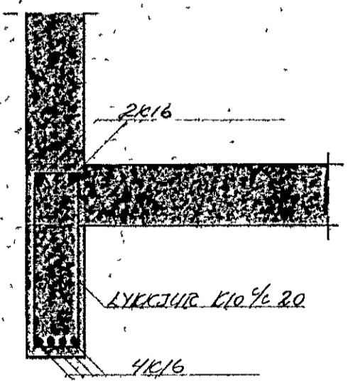
BITI B-1 VFR GLÖGGUM L=45 1:20
