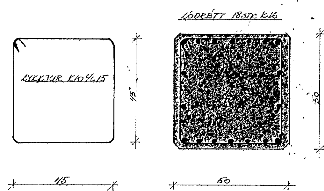
SÚLA 5-1 1:10
