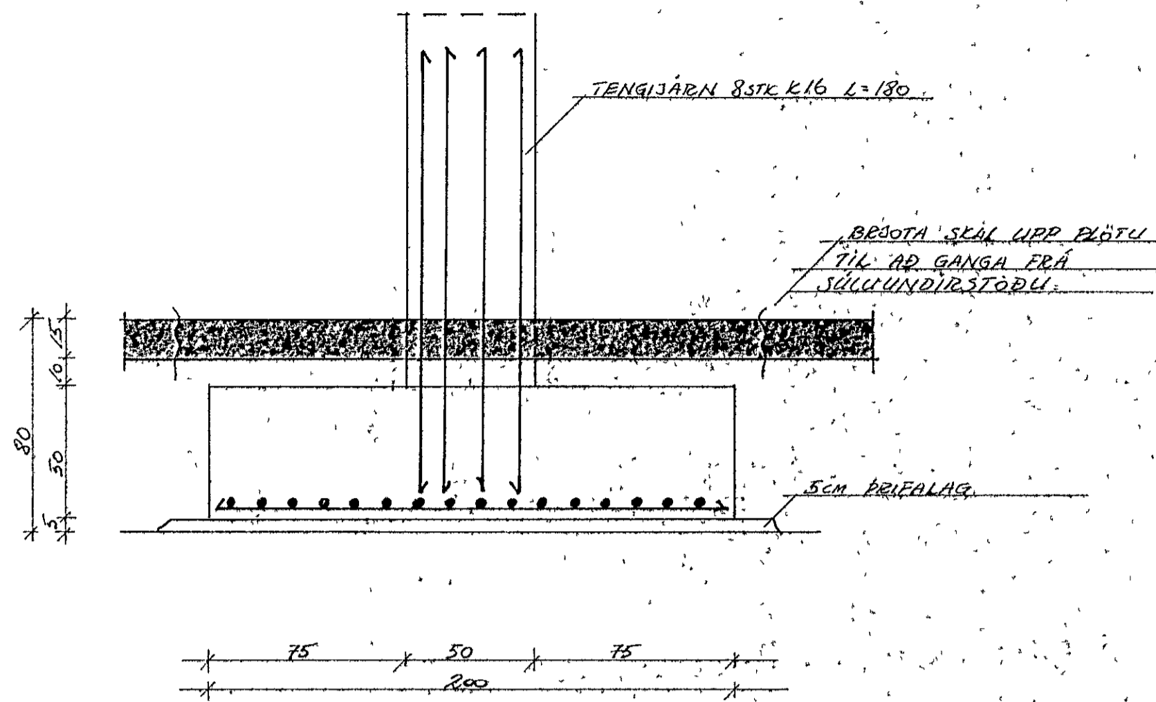
UNDIRSTÖÐA 1-1 1:20
