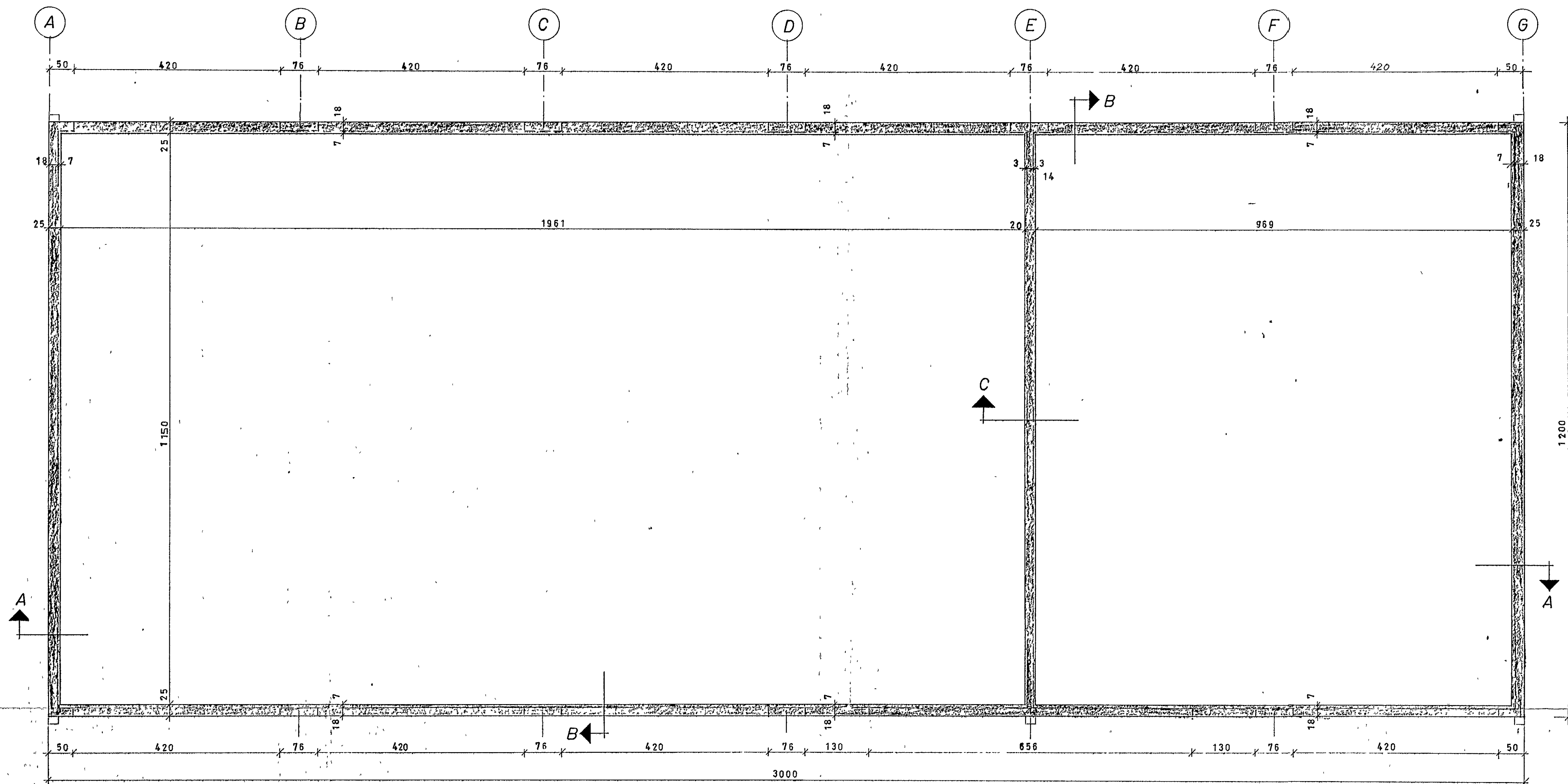
GRUNNMYND - UNDIRSTÖÐUR 1:50
