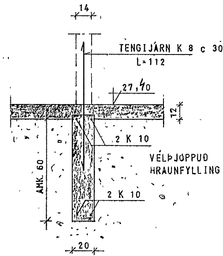
SNÍÐ C 1:20
