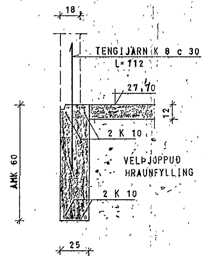
SNÍÐ A 1:20
