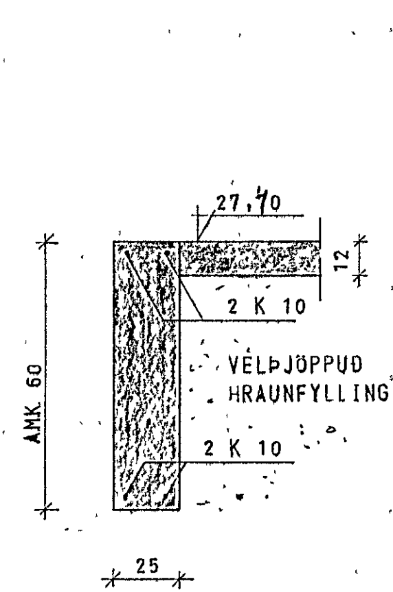
SNÍÐ B 1:20
