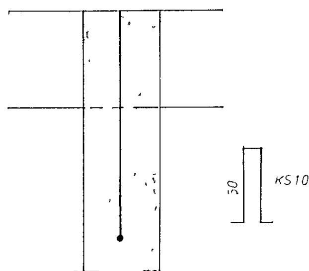
F3 m=1:10
