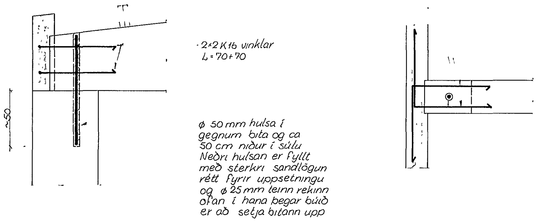
FRÁGANGUR BITAFESTINGA 1:20
