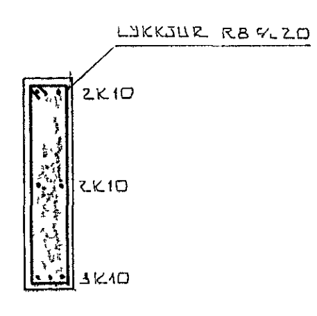
SNID B-B ~ 1:20
