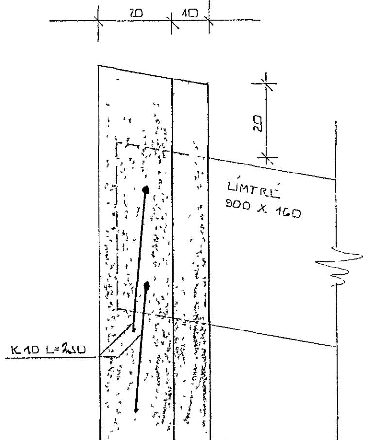
SNID E ~ 1:10
