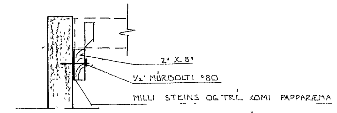
SNID D - D ~ 1:20
