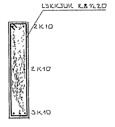
SNID C-C ~ 1:20
