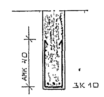
SNID A-A ~ 1:20
