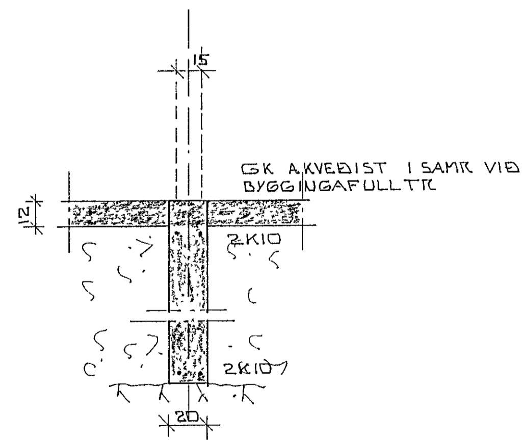
SNIÐ Í INNVEGG 1:20
