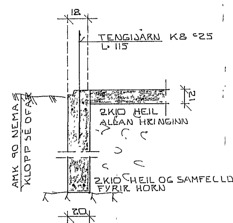
SNIÐ Í ÚTVEGG 1:20
