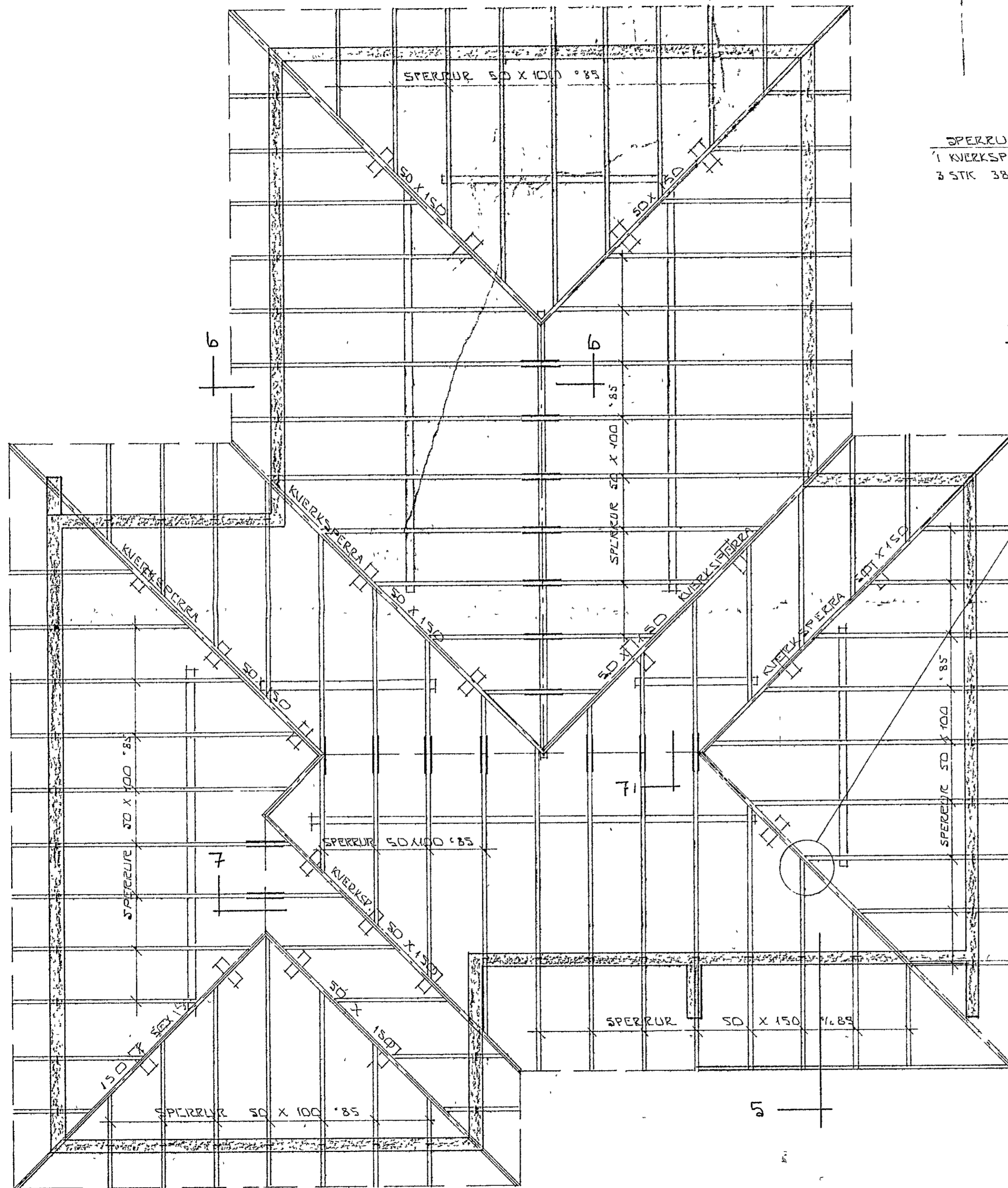
GRUNNMYND 1:50
