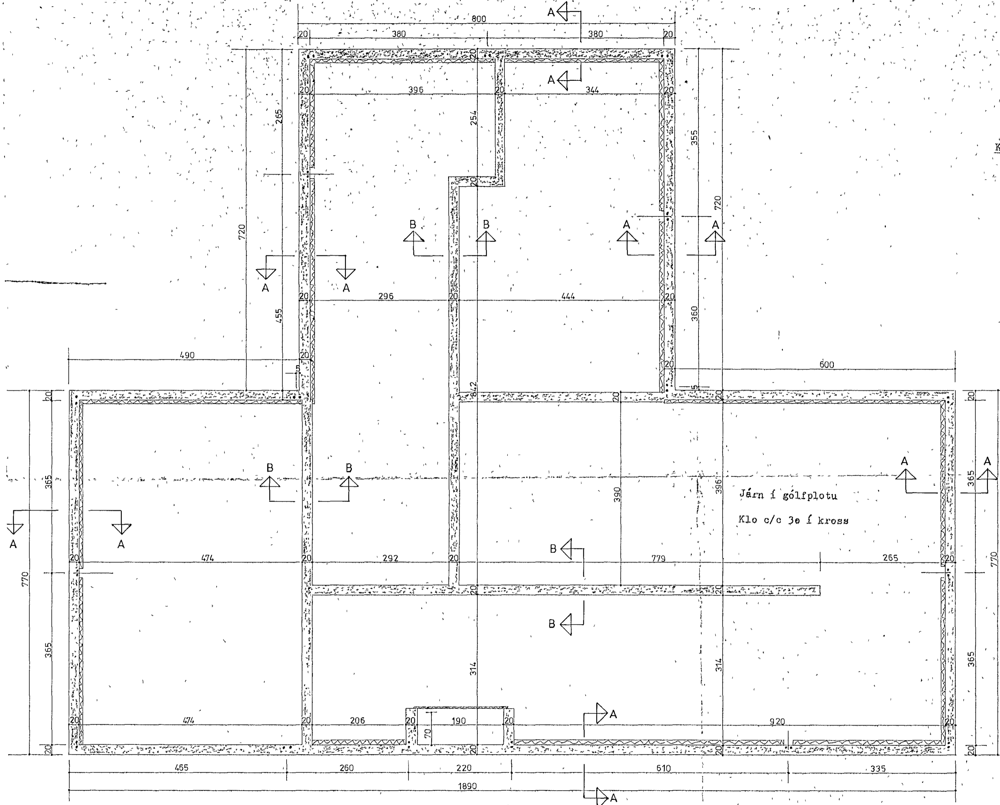
GRUNNMYND M: 1:50
