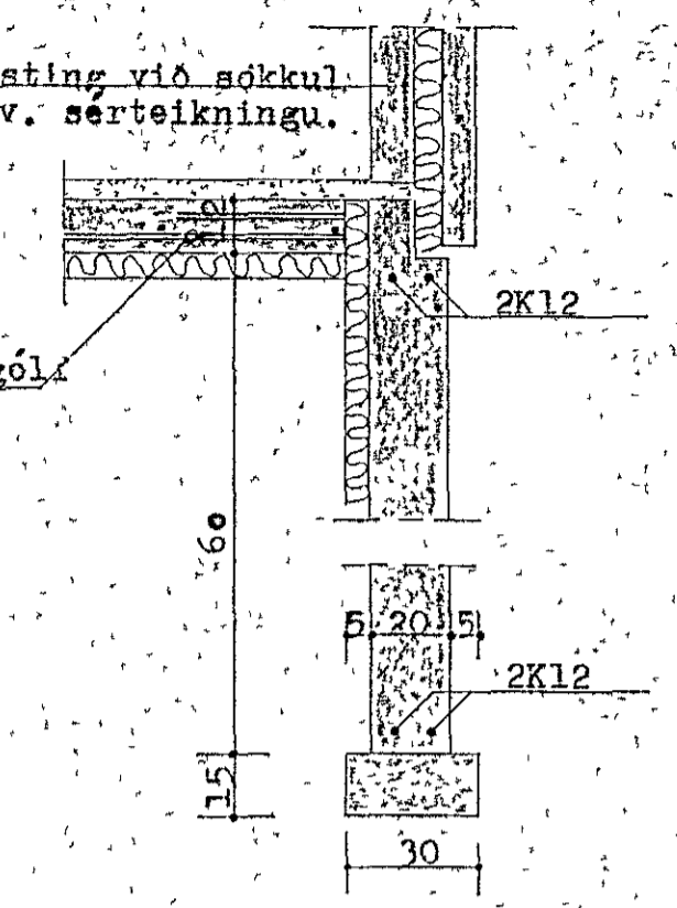
SNÍÐ A-A M: 1:20
