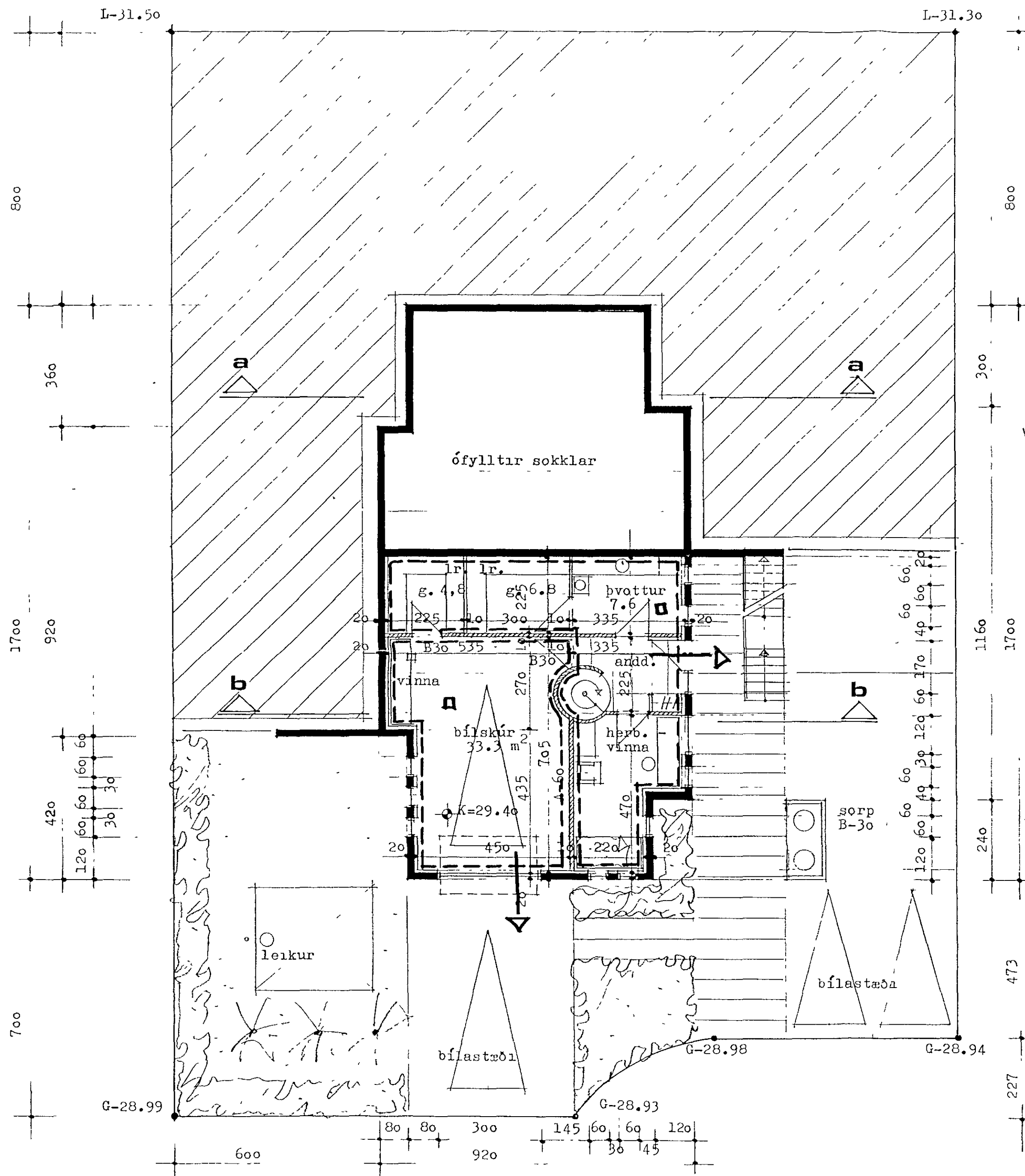
jarðhæð - grunnmynd 1:100
