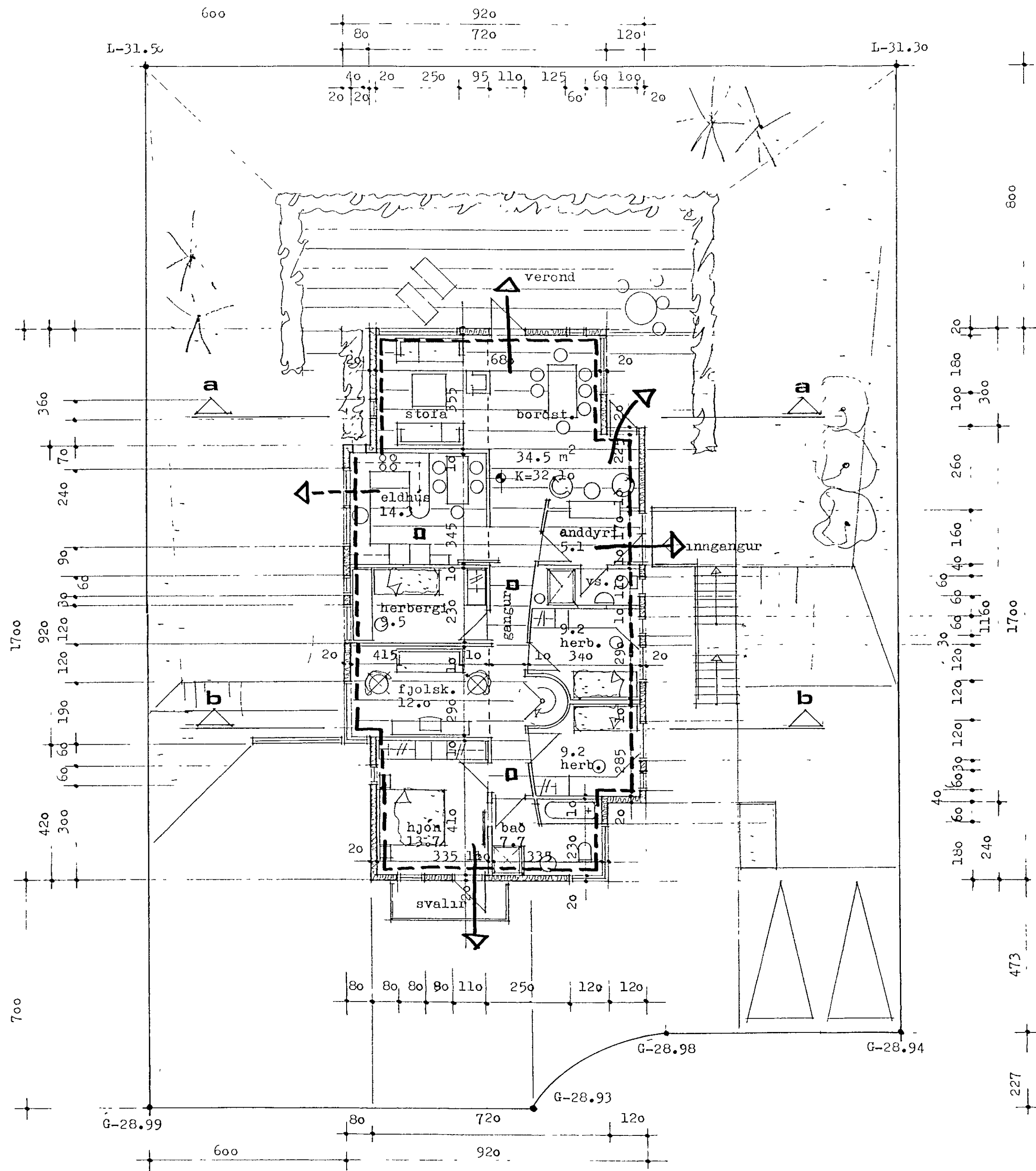
efri hæð - grunnmynd 1:100
