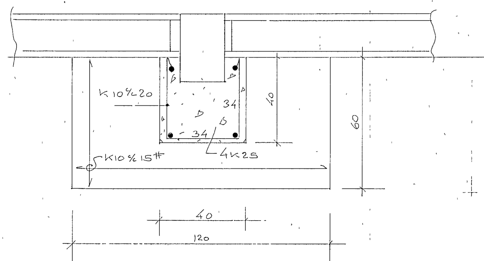
SÚLUFÓTUR 1:10
