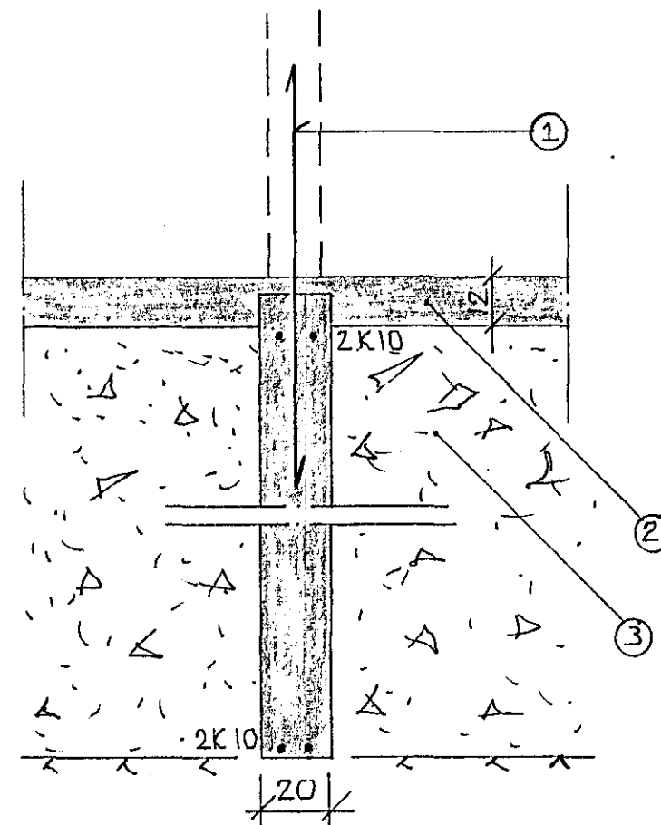
SNID 3 Í MILLVEGGI • 1:20
