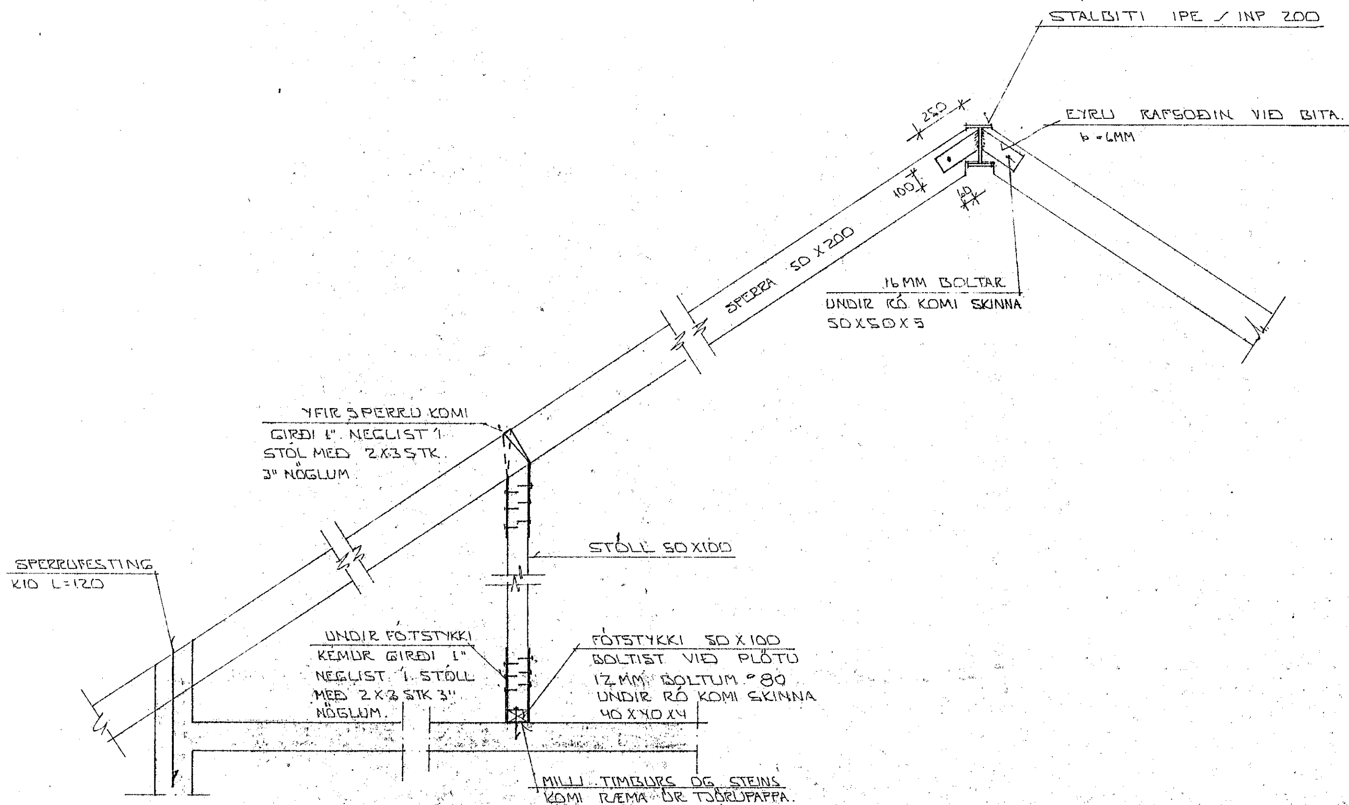
SNIED 5 - 5 í ÞAK 1:20
