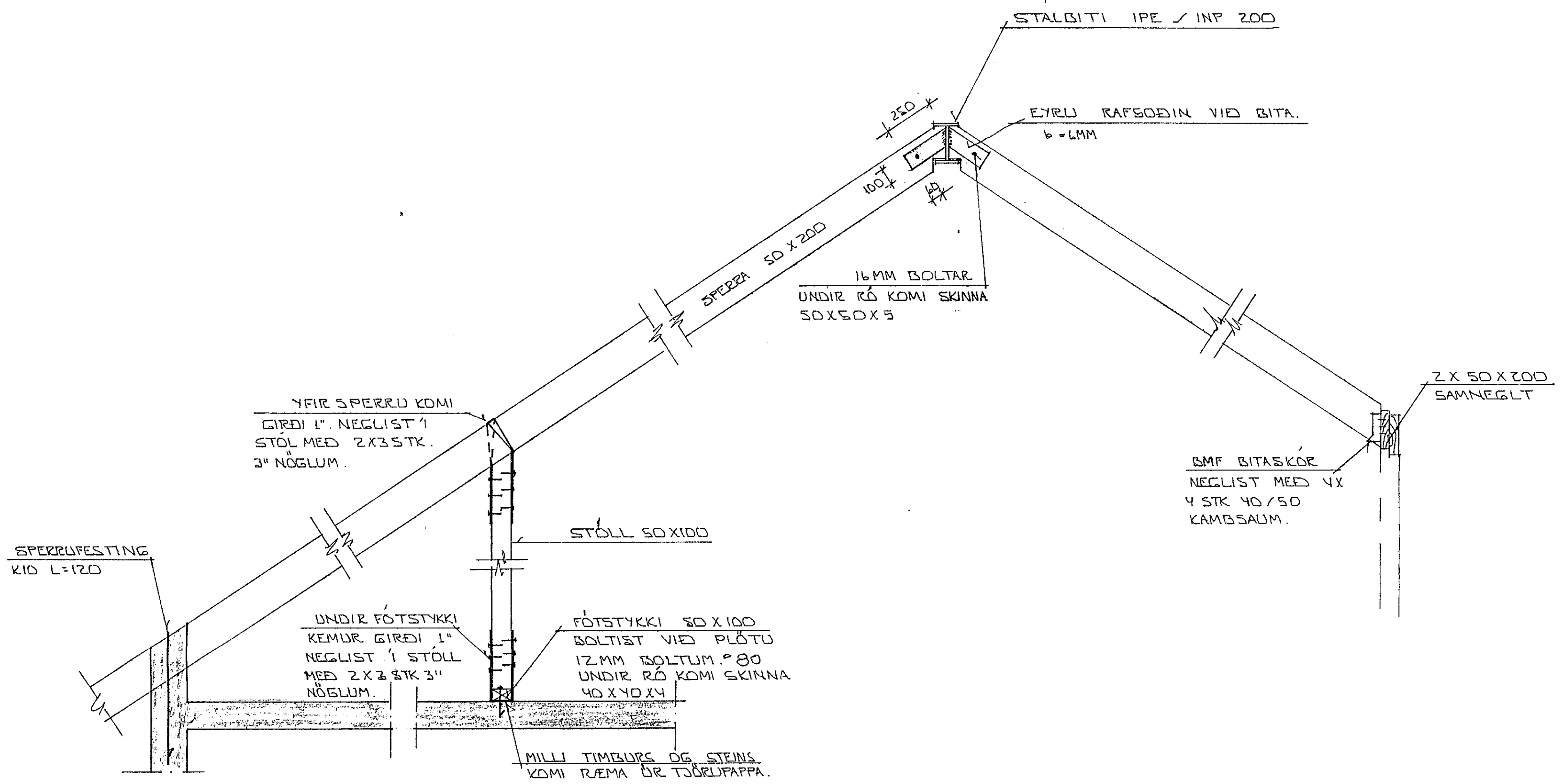
SNÍÐ 3 - 3 Í ÞAK 1:20
