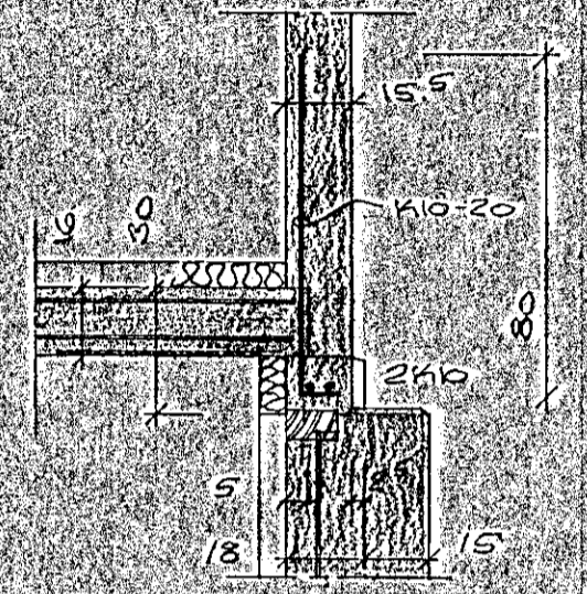
SKURÐUR A-M:1:20
