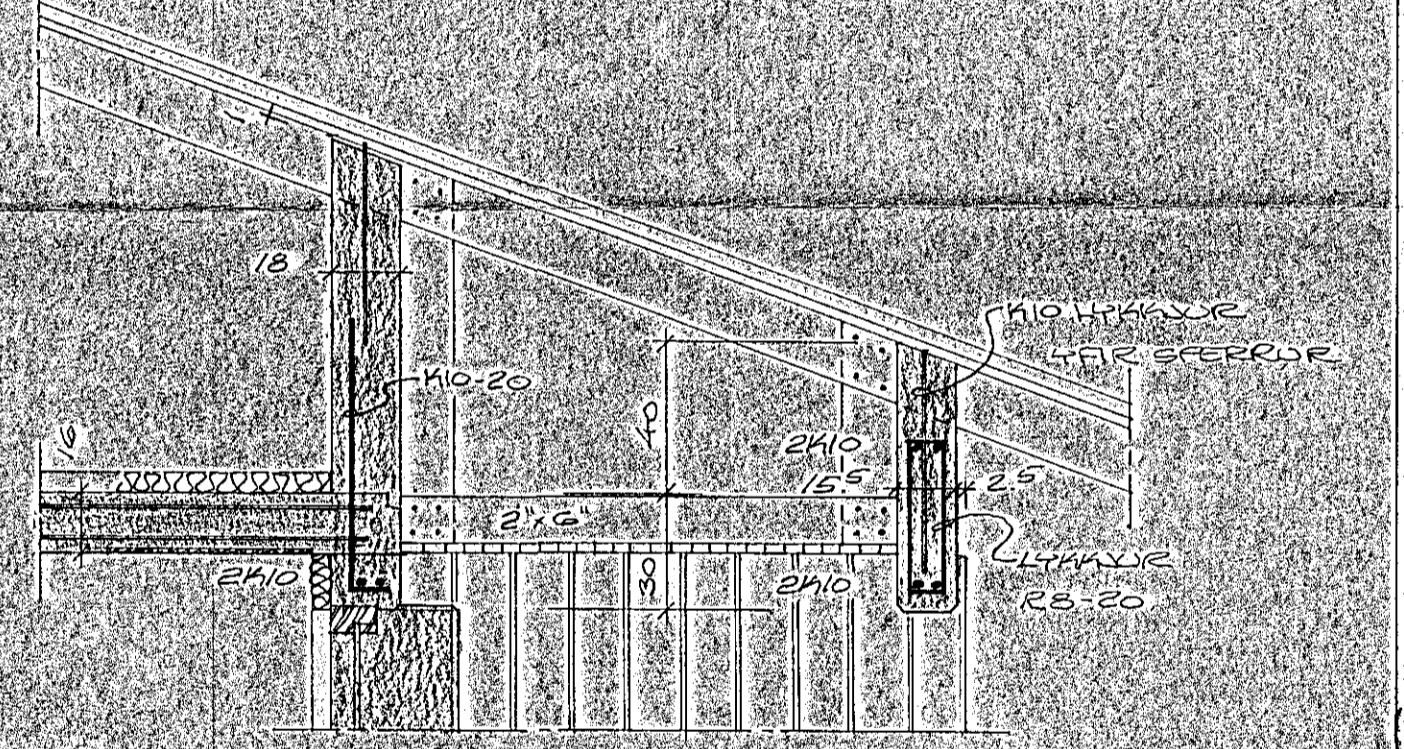
SKURÐUR C-M:1:20
