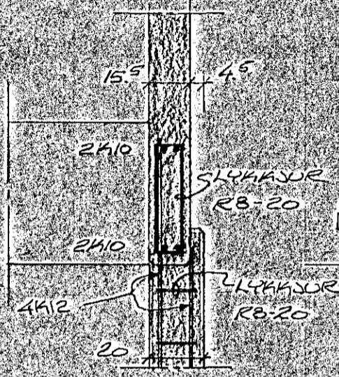
SKURÐUR E-M:1:20
