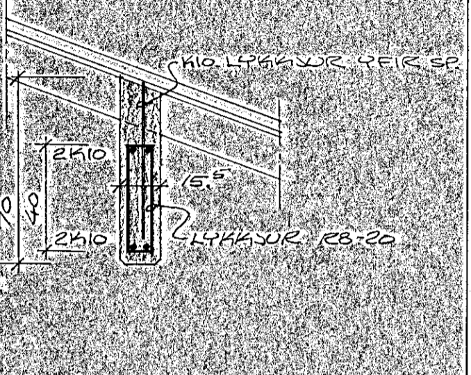
SKURÐUR D-M:1:20
