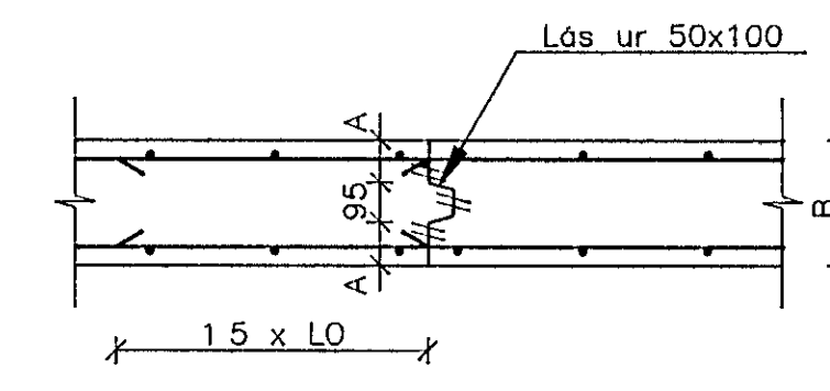
10 SNID 102 M. 1:20
