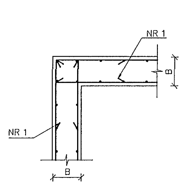
1 SNID 102 M. 1:20
