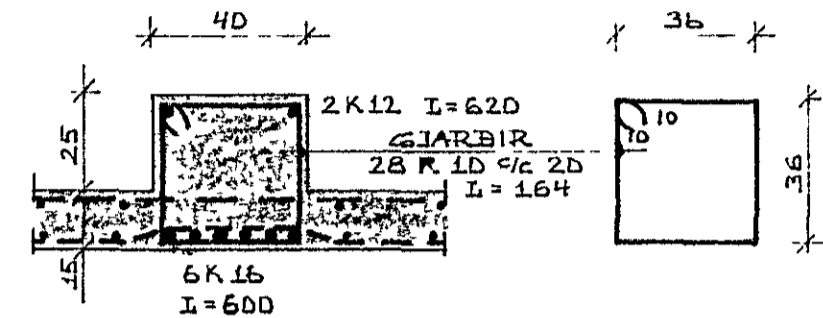
SNID A-A 1:20
