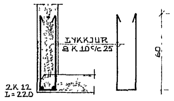
SNID D-D 1:20
