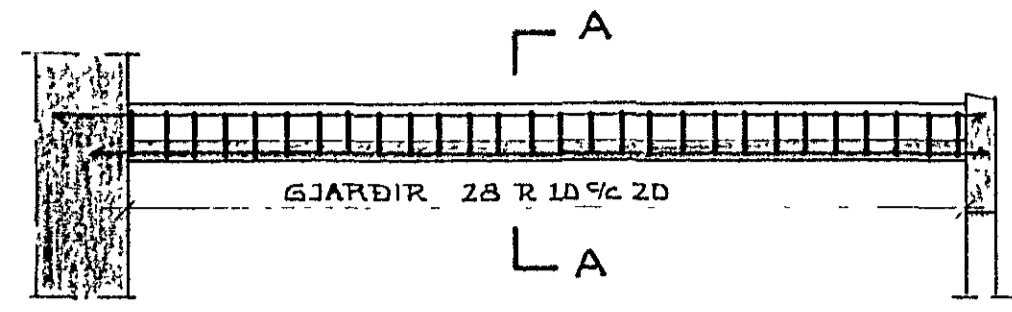
BITI B1 1:50
