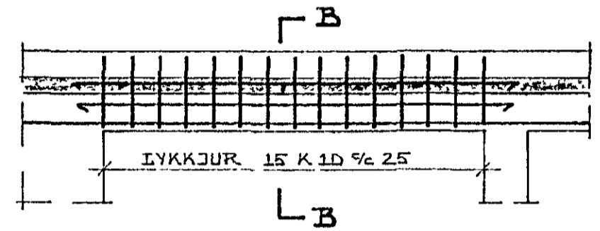
BITI B2 1:50
