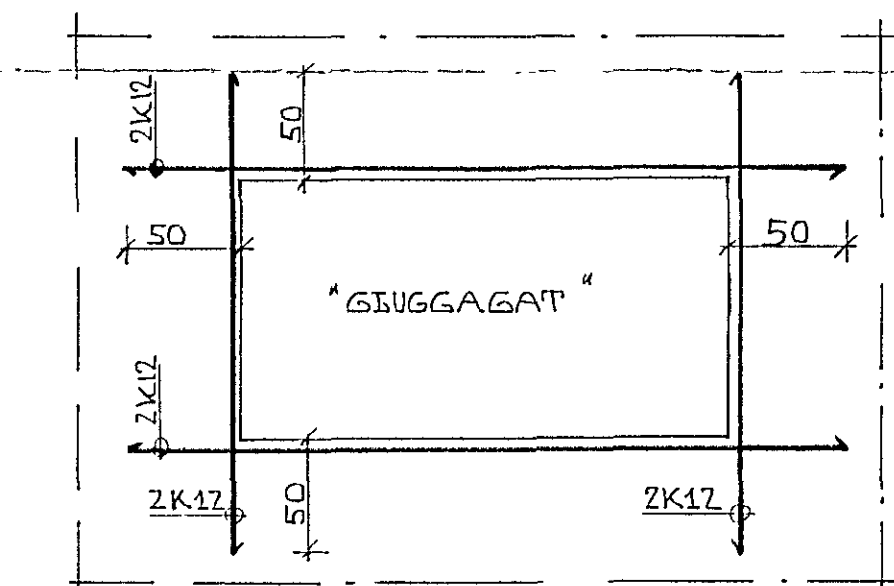
BÁRETT SNIÐ
