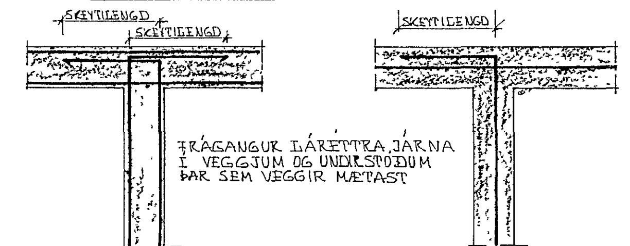
BÁRETT SNIÐ
