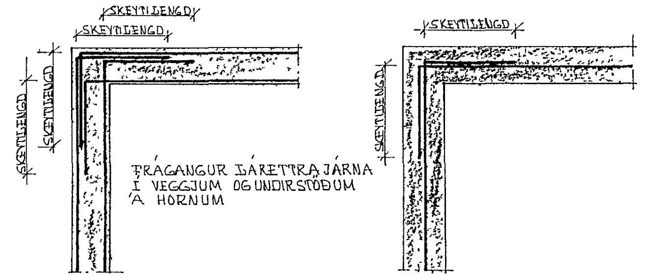
LÁRETT SNIÐ
