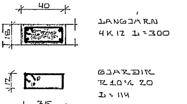
SNID Í SÚLU S2 1:20
