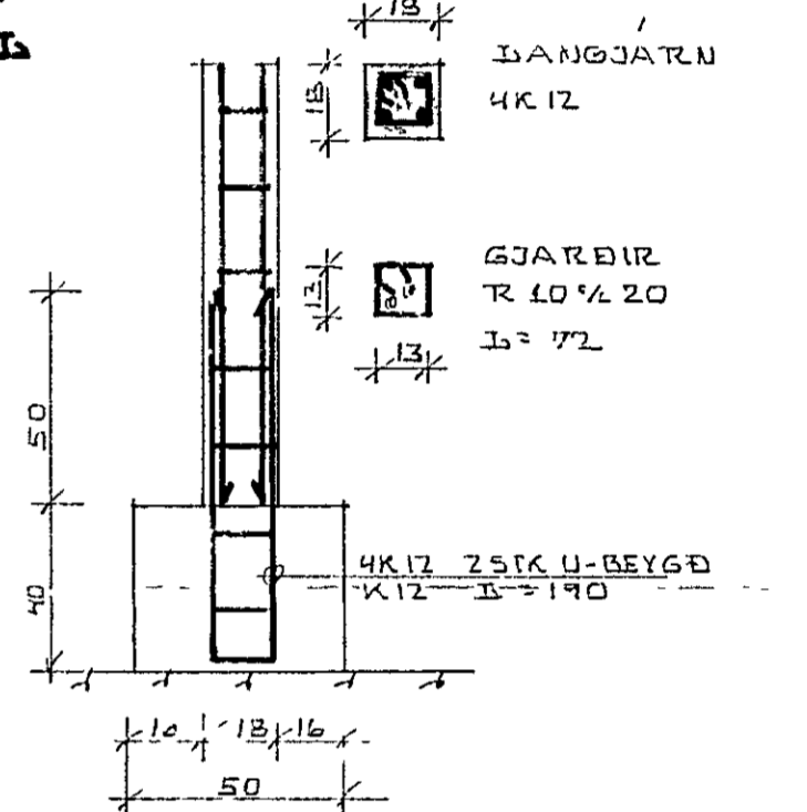
SÚLA S4 1:20
