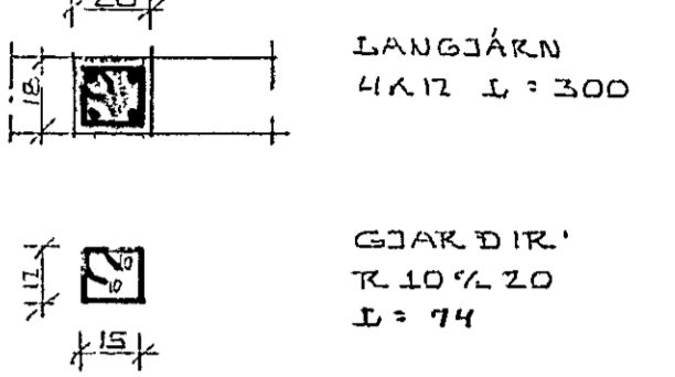
SNID Í SÚLU S1 1:20
