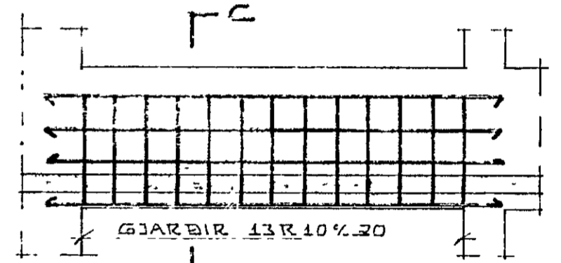
SNIB B-B 1:50
