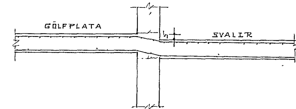
SKURÐUR I GÖLFPLÖTU OG SVALIR KVARDI 1/20
