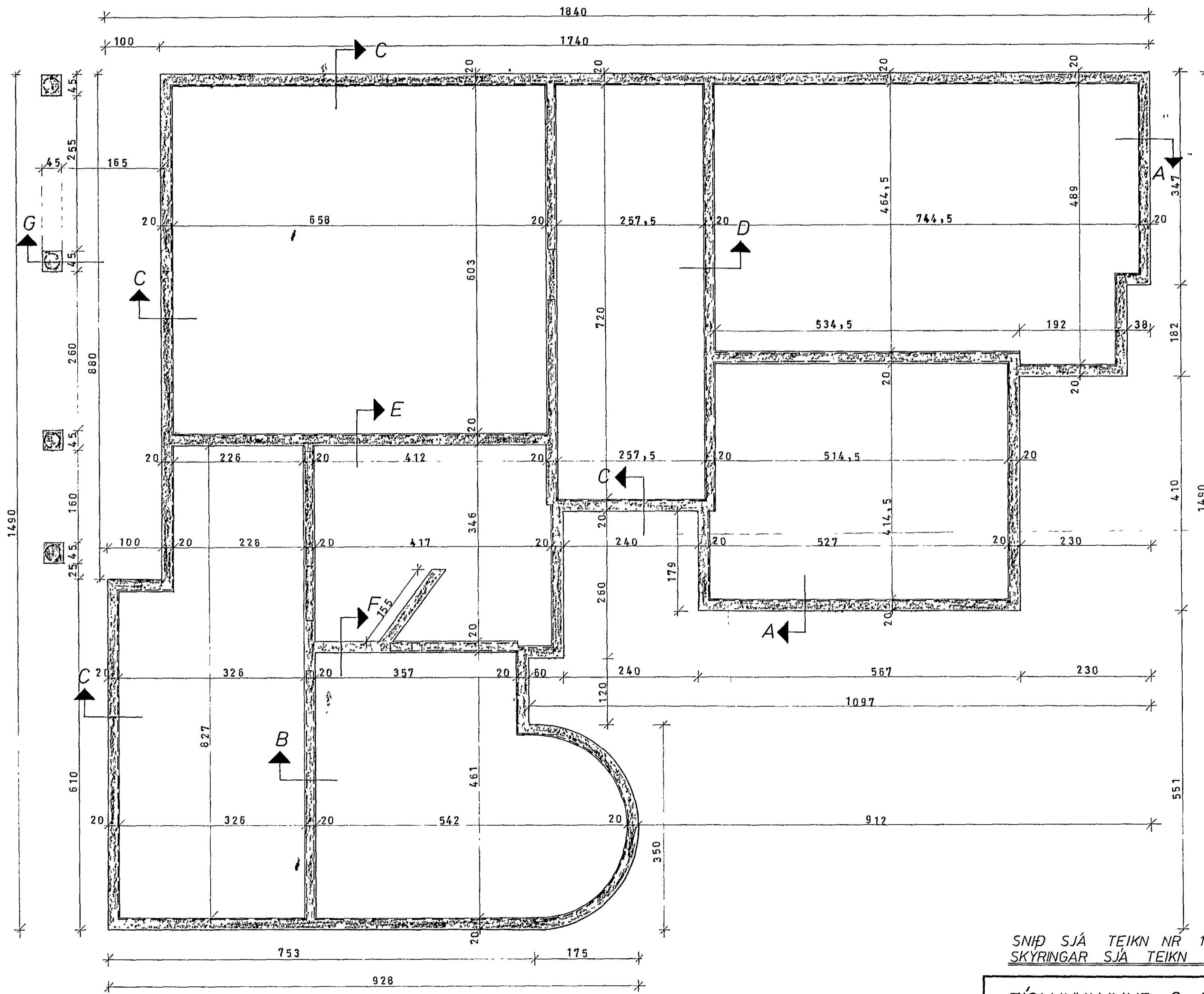
GRUNNMYND - UNDIRSTOÐUR 1:50
