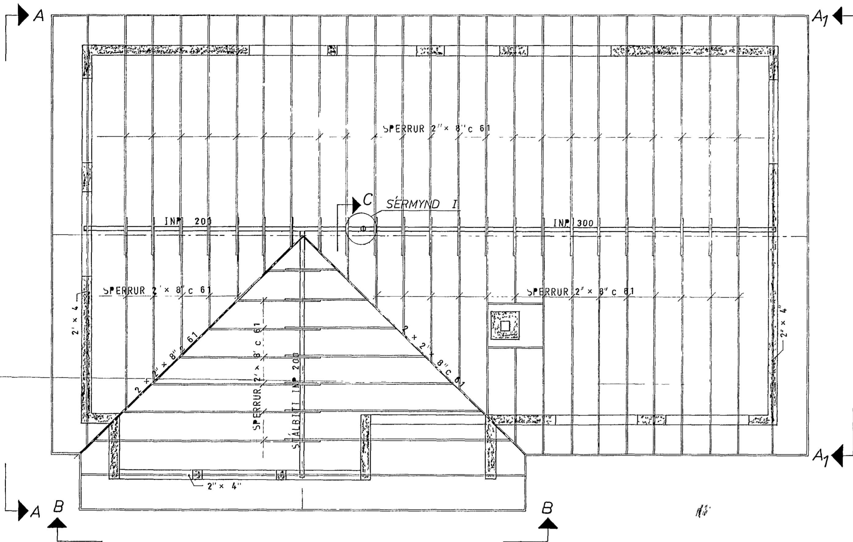
GRUNNMYND 1 50
