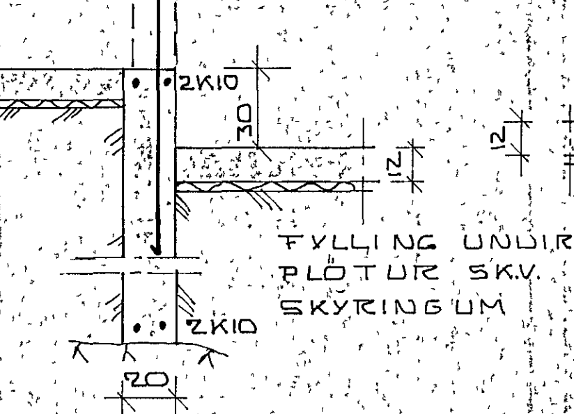
SNID D-D
