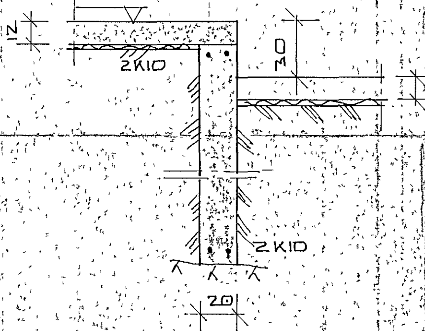
SNID I-I
