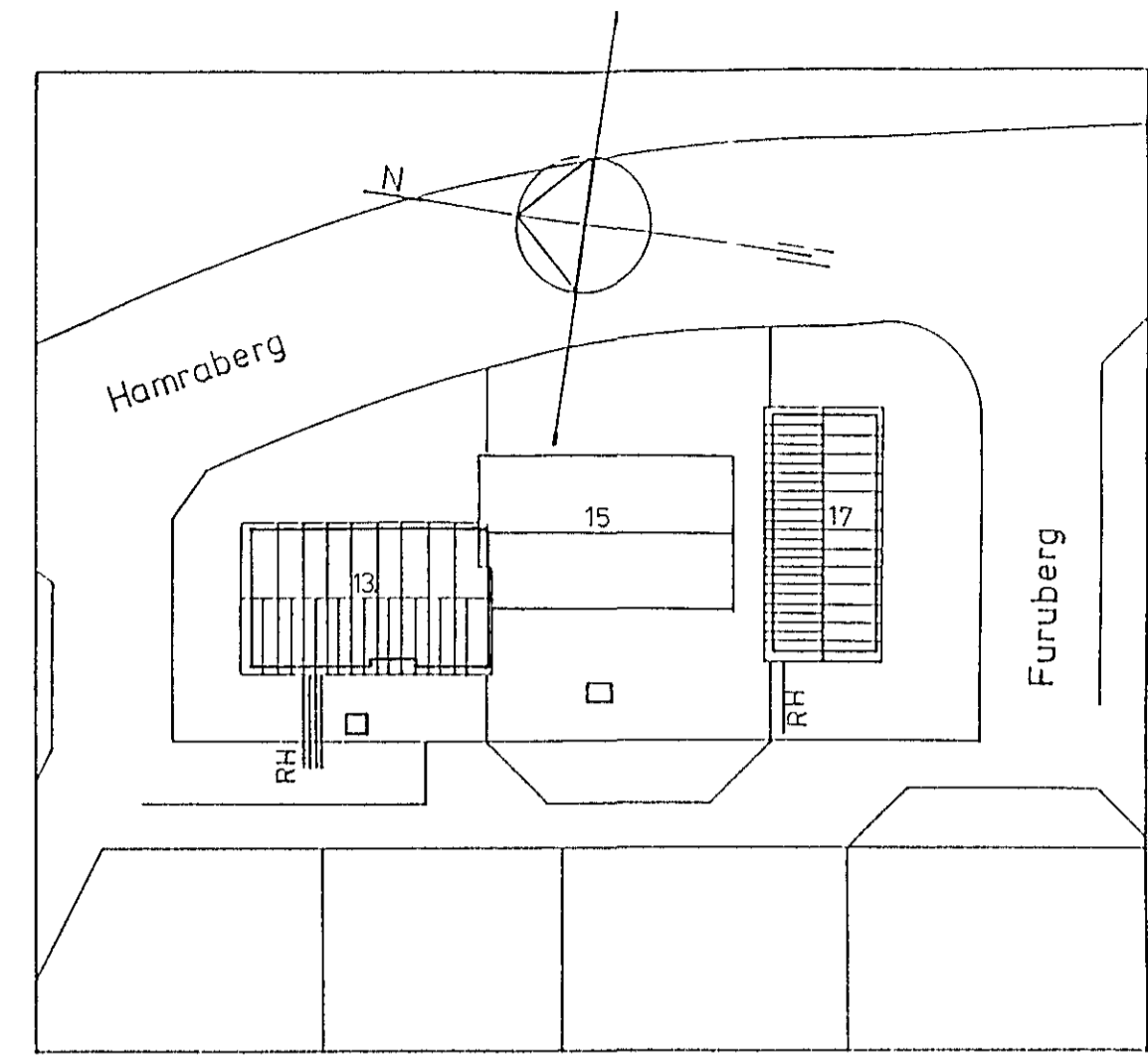
AFSTÖÐUMYND 1 500
