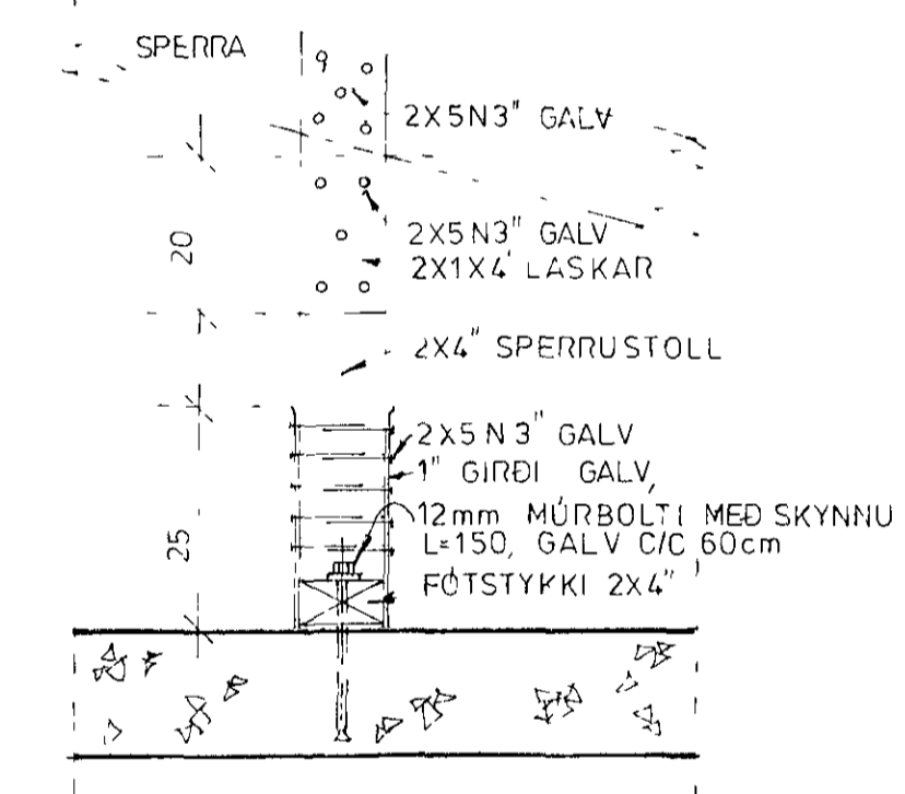
SNIÐ B- (FRÁGANGUR A STÖLUN VIÐ SPERRUR)
