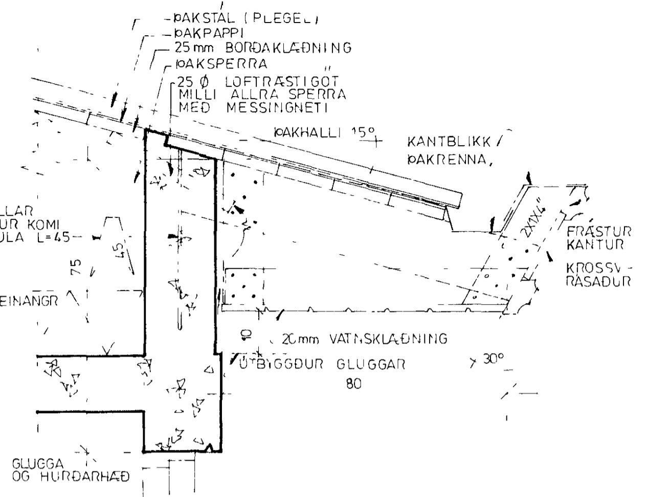
SNIÐ A- (FRÁGANGUR VIÐ ÞAKKANT OG ÞAK)
