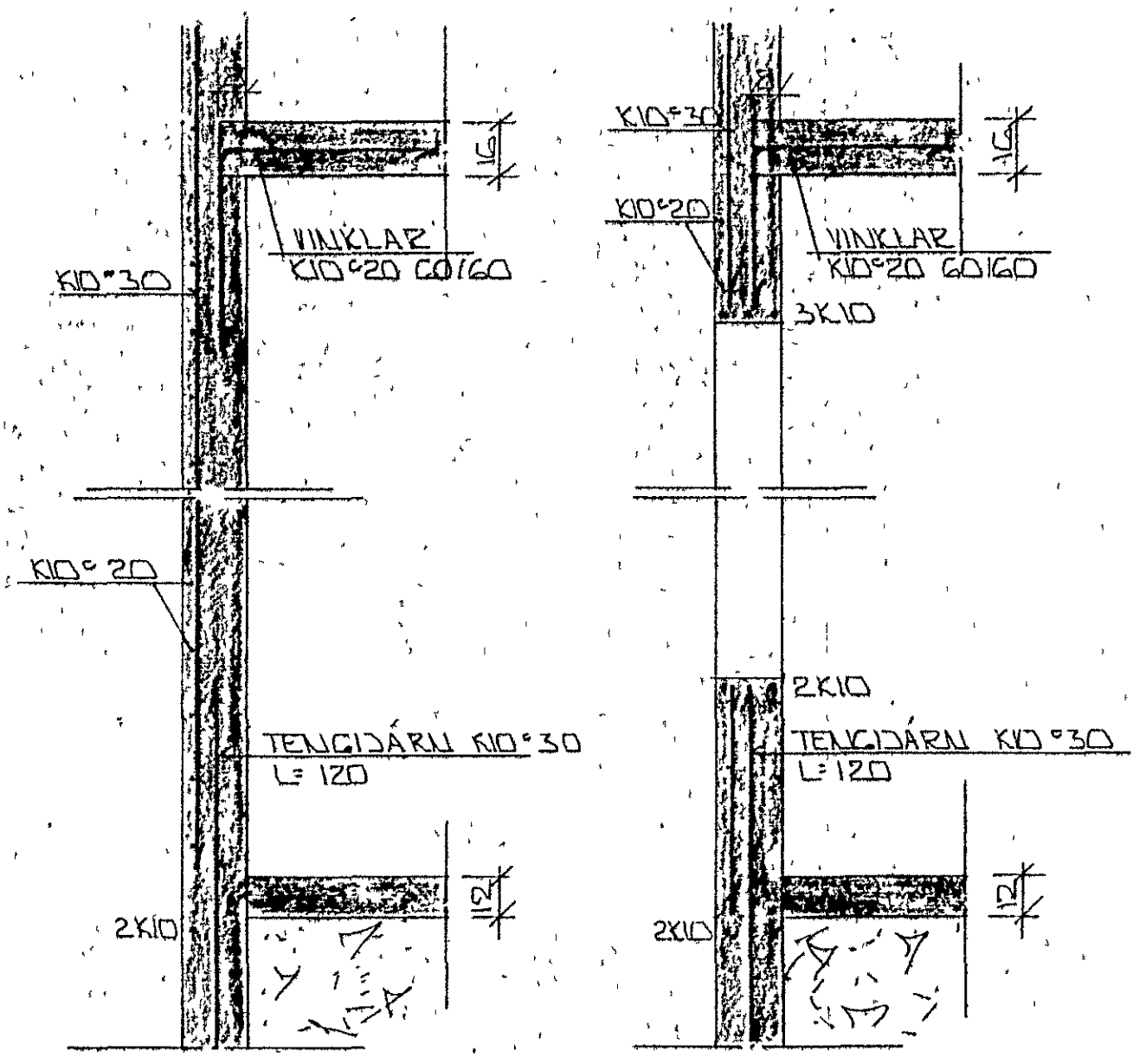
SNID X · 1:20
