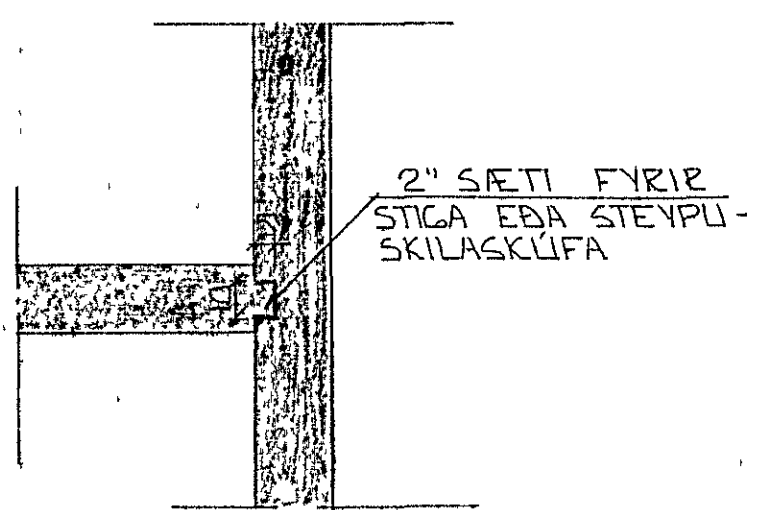
SNID 9 · 1:20
