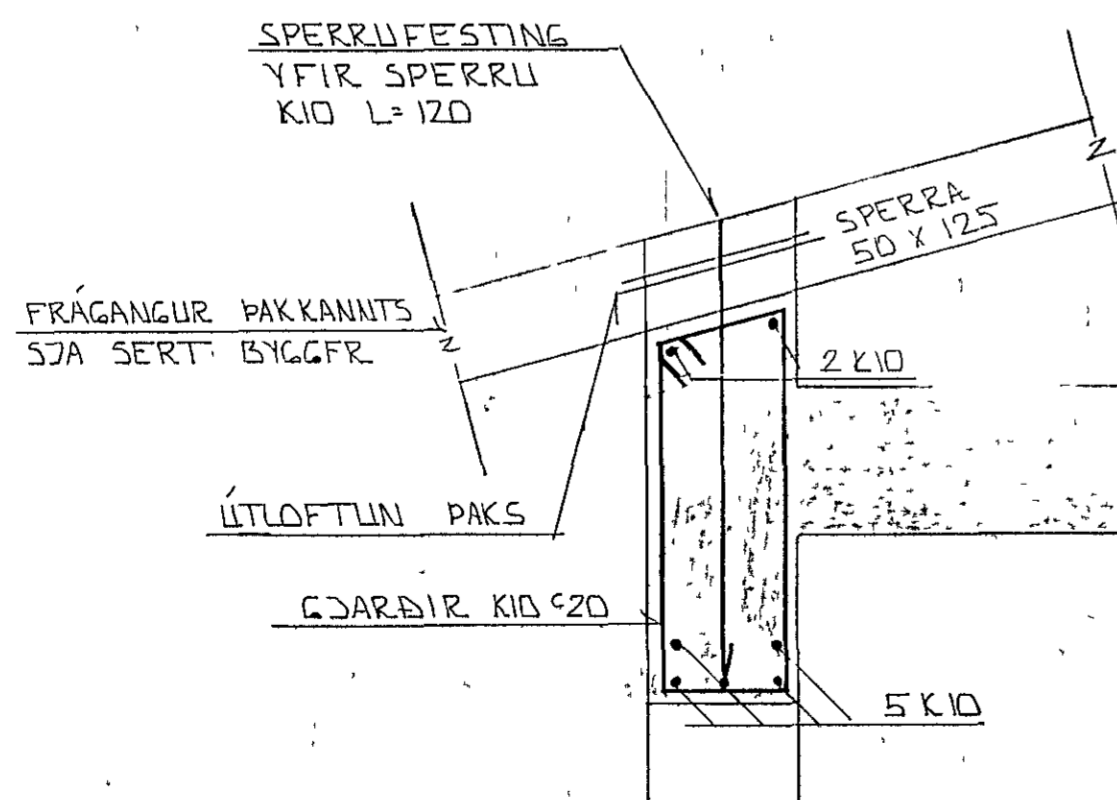
SNID 8 YFIR SVALAGLUGGUM • 1:10
