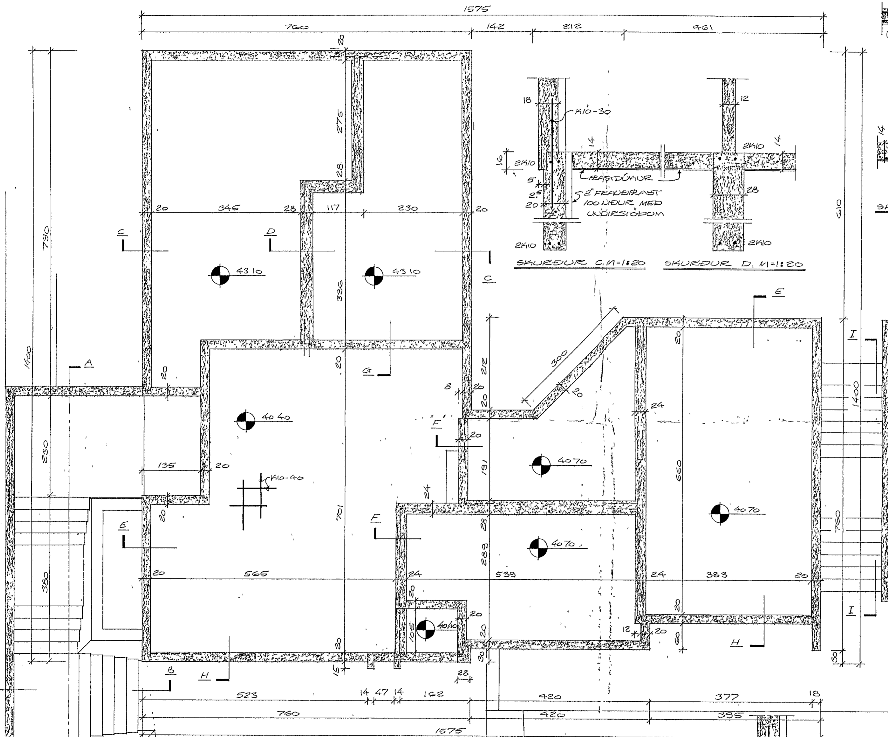
GRUNNMYND, M=1:50
