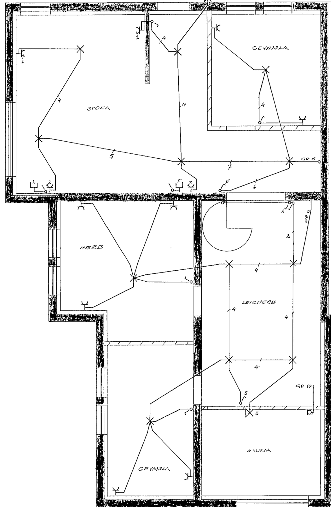
RAFLOGU KJALLARA 1 50
