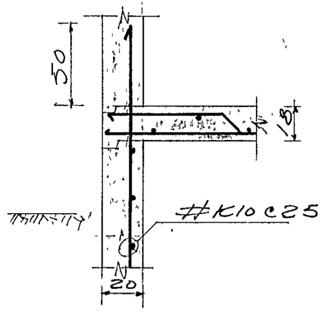
SNID A-A 1:20
