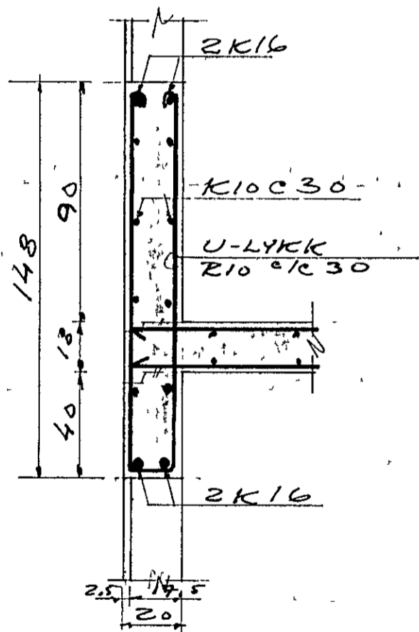
SNID B-B 1:20
