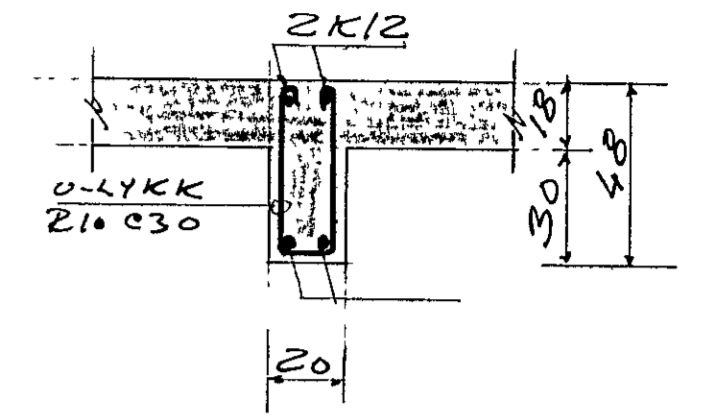
SNID D-D 1:20
