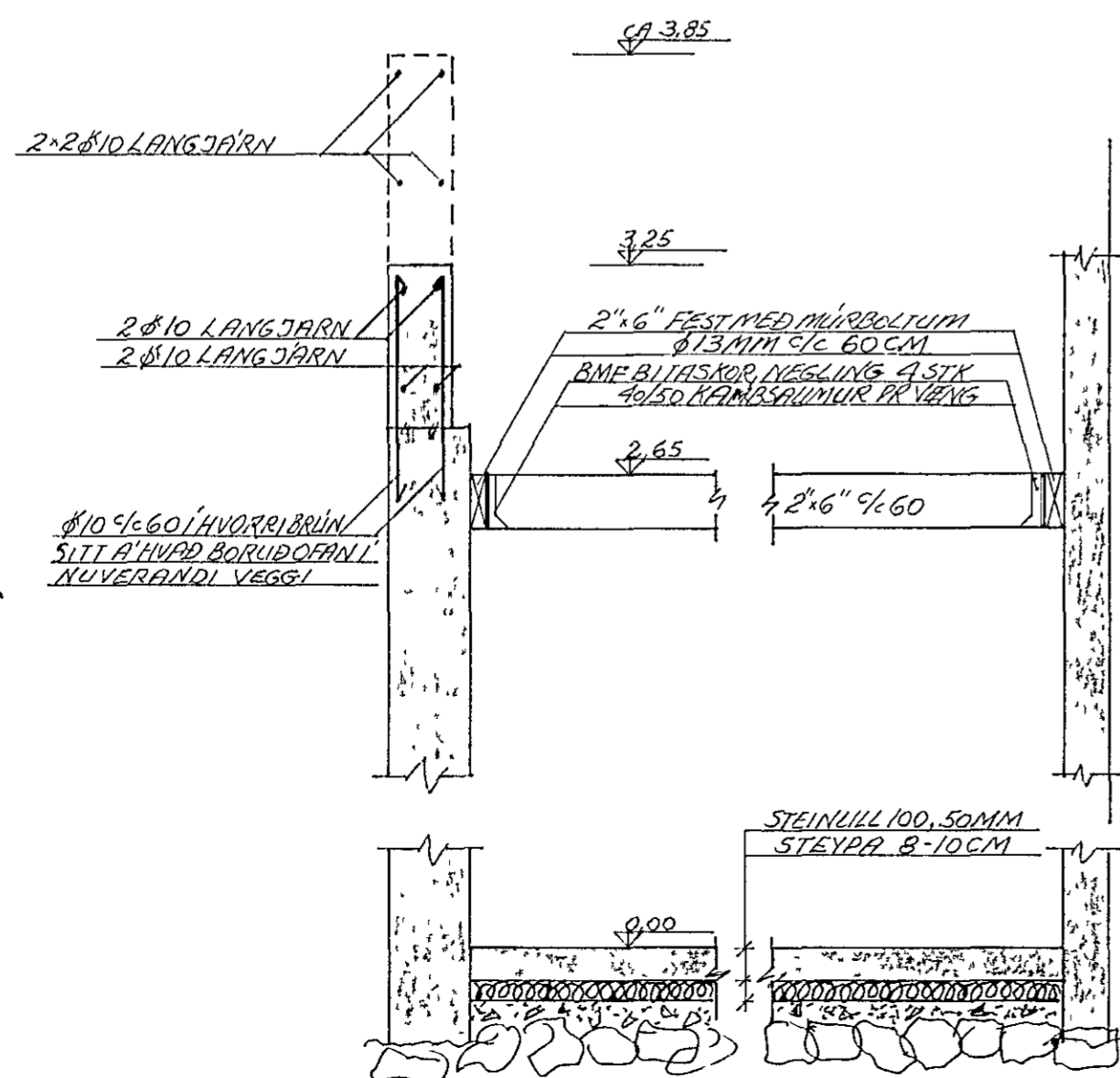
SNID 1-1 1:20
