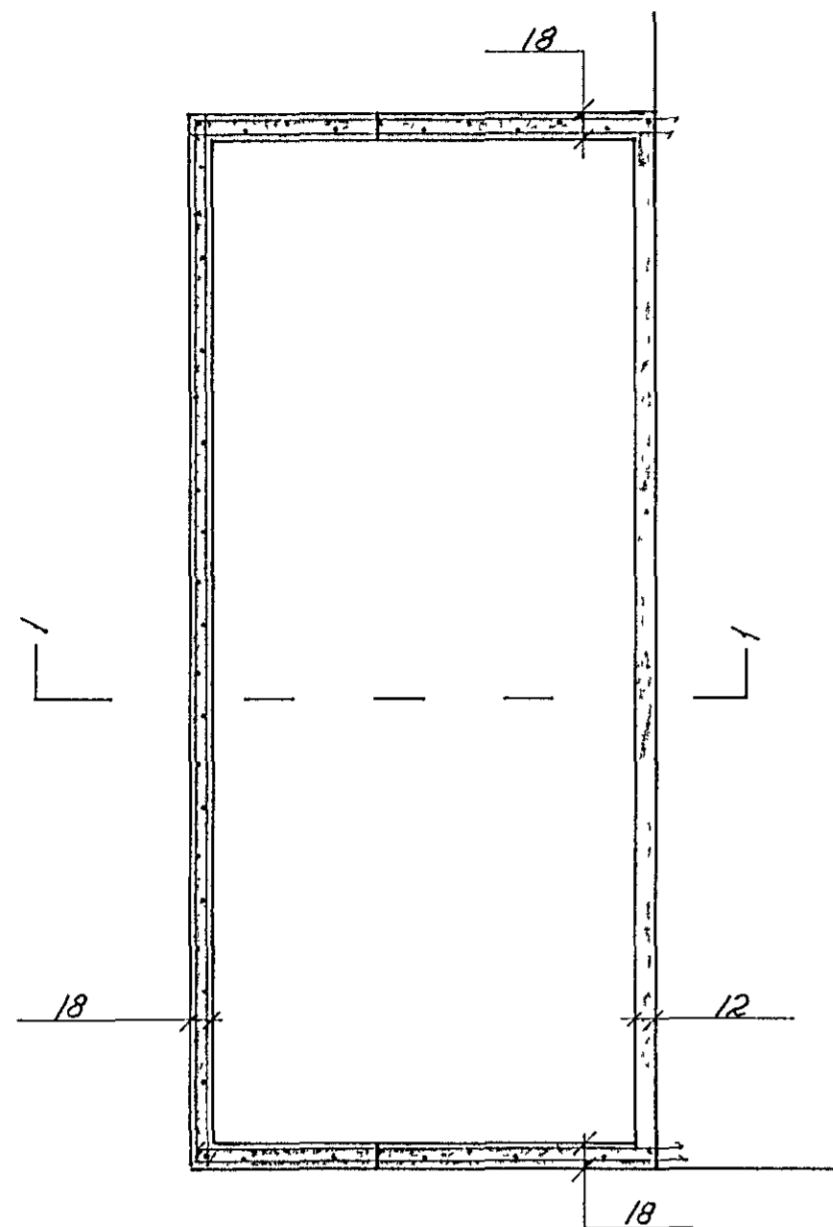
VEGGIR GRUNNMYND 1:50
