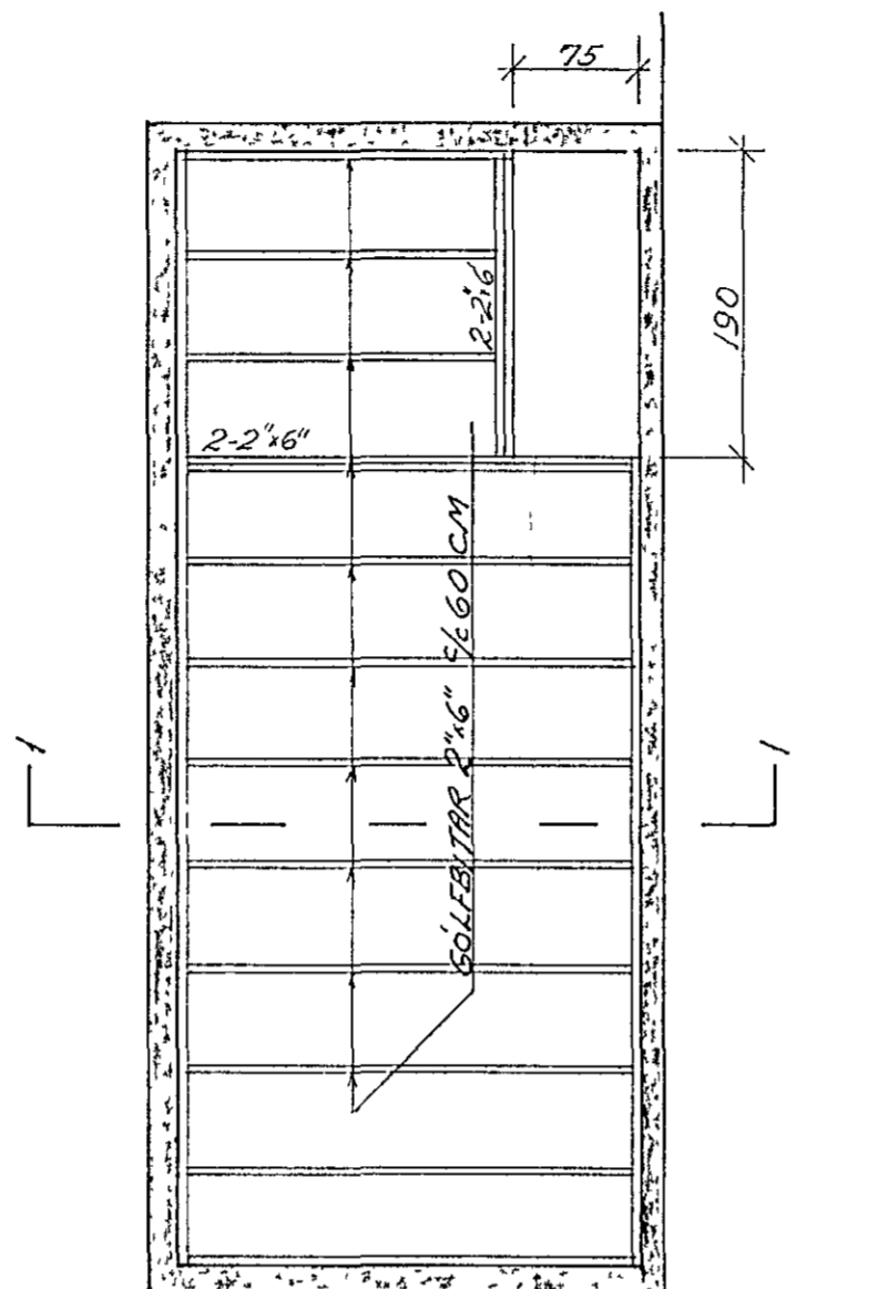
GÓLF GRUNNMYND 1:50
